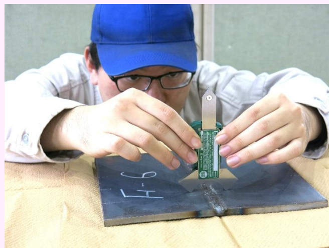
外観試験
