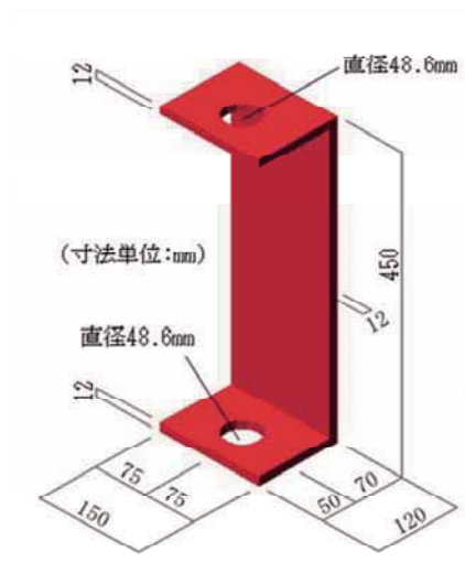
図 3-18 治具の寸法
