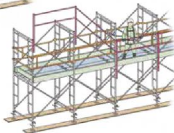
わく組足場
