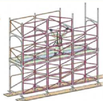
わく組足場
