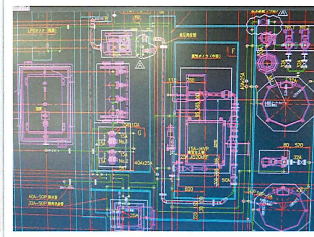
【当社作成 施工图】
