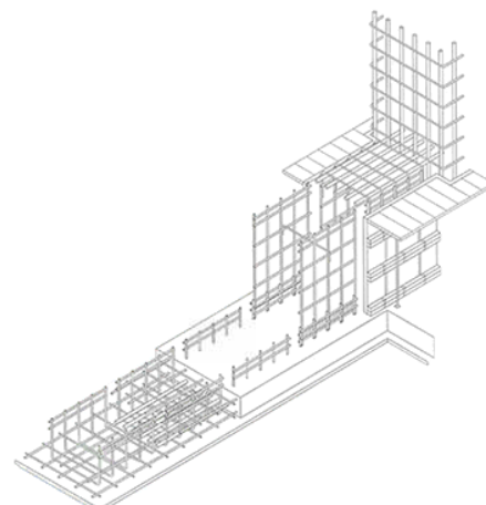
二線溶接工法（二線メッシュ工法）
