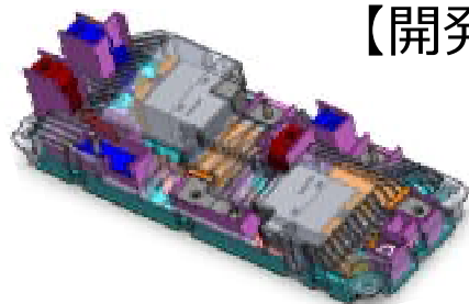
【高圧ジャンクションブロック】 電動車の電源分配・遮断BOX
