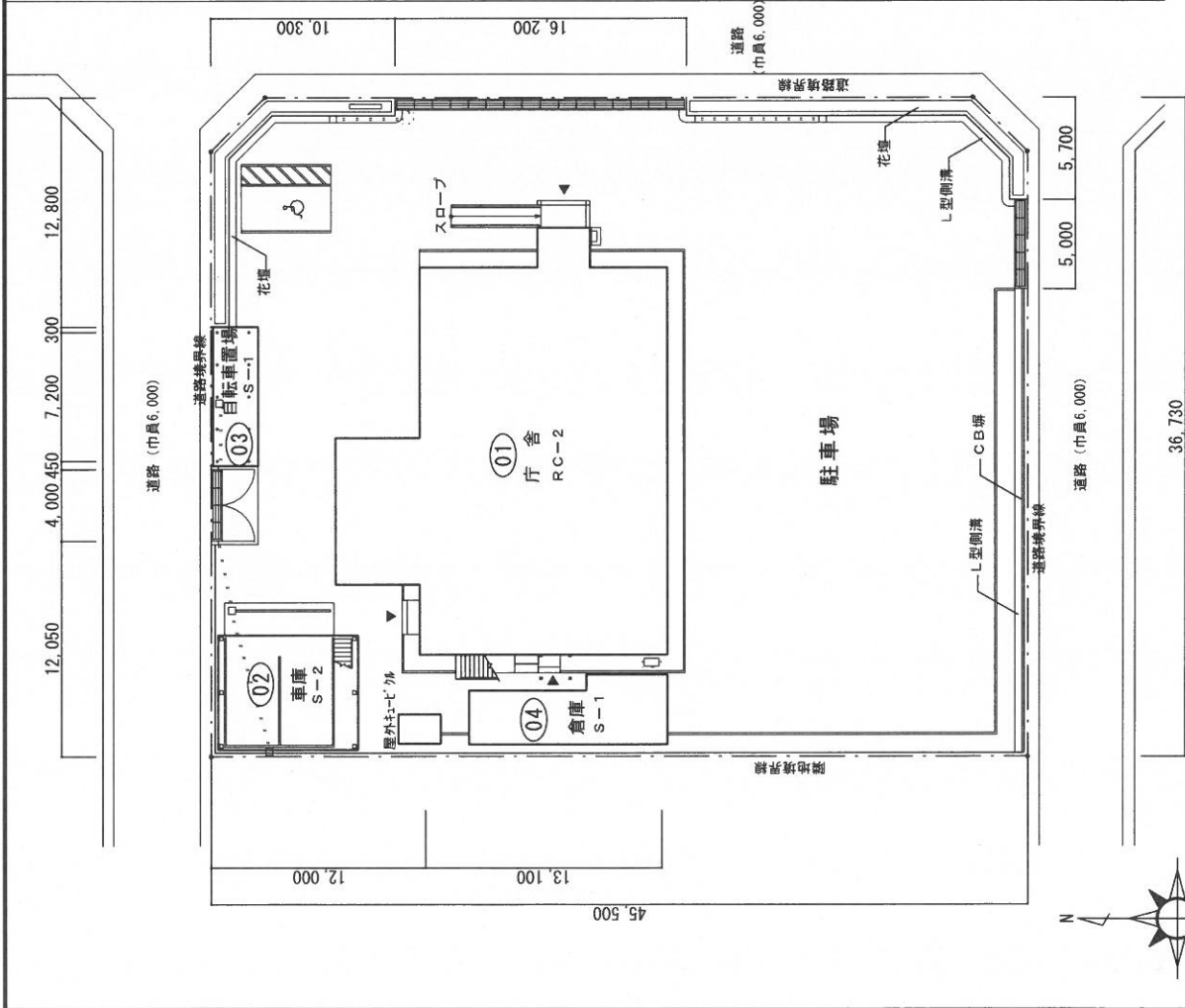
配置図 S=1/400
