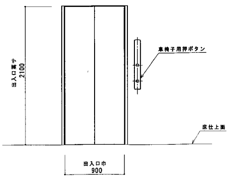
乗場正面図 (1/20) (1FL)
