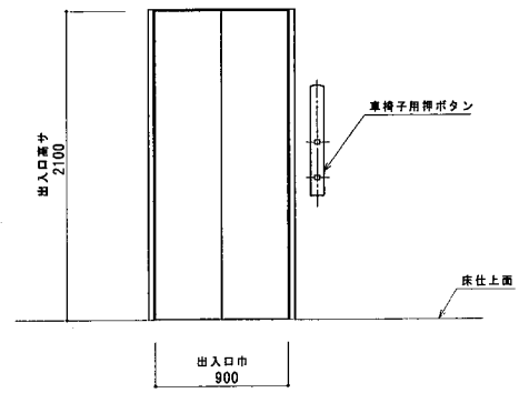
乗場正面図 (1/20) (2FL)
