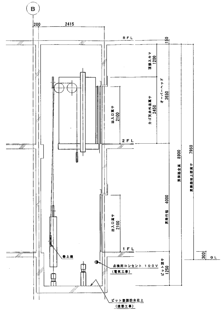
昇降路縦断面図 (1/30)
