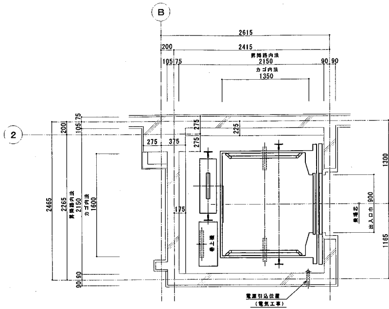
昇降路平面図 (1/20) (1・2FL)
