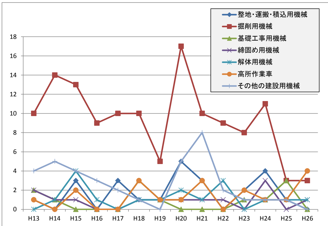
図2 建設用機械に起因した労働災害の起因物(小分類)別内訳
