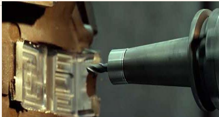
加工の様子
