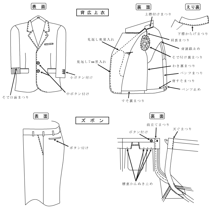
男子既製洋服のまとめ業務工程解説図
