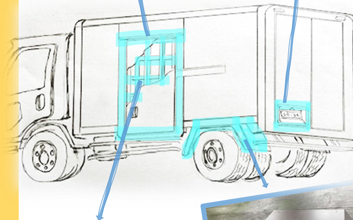
宅配トラック 扉本体骨組み
