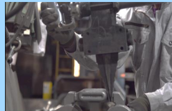
④製品がコンベアで流れてくるので、工具等を使い切り離していきます。周りについている砂なども取りきれいにします。
