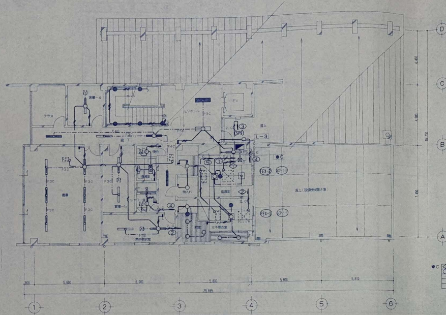
3階 電灯（照明）設備配線図 S=1:100
