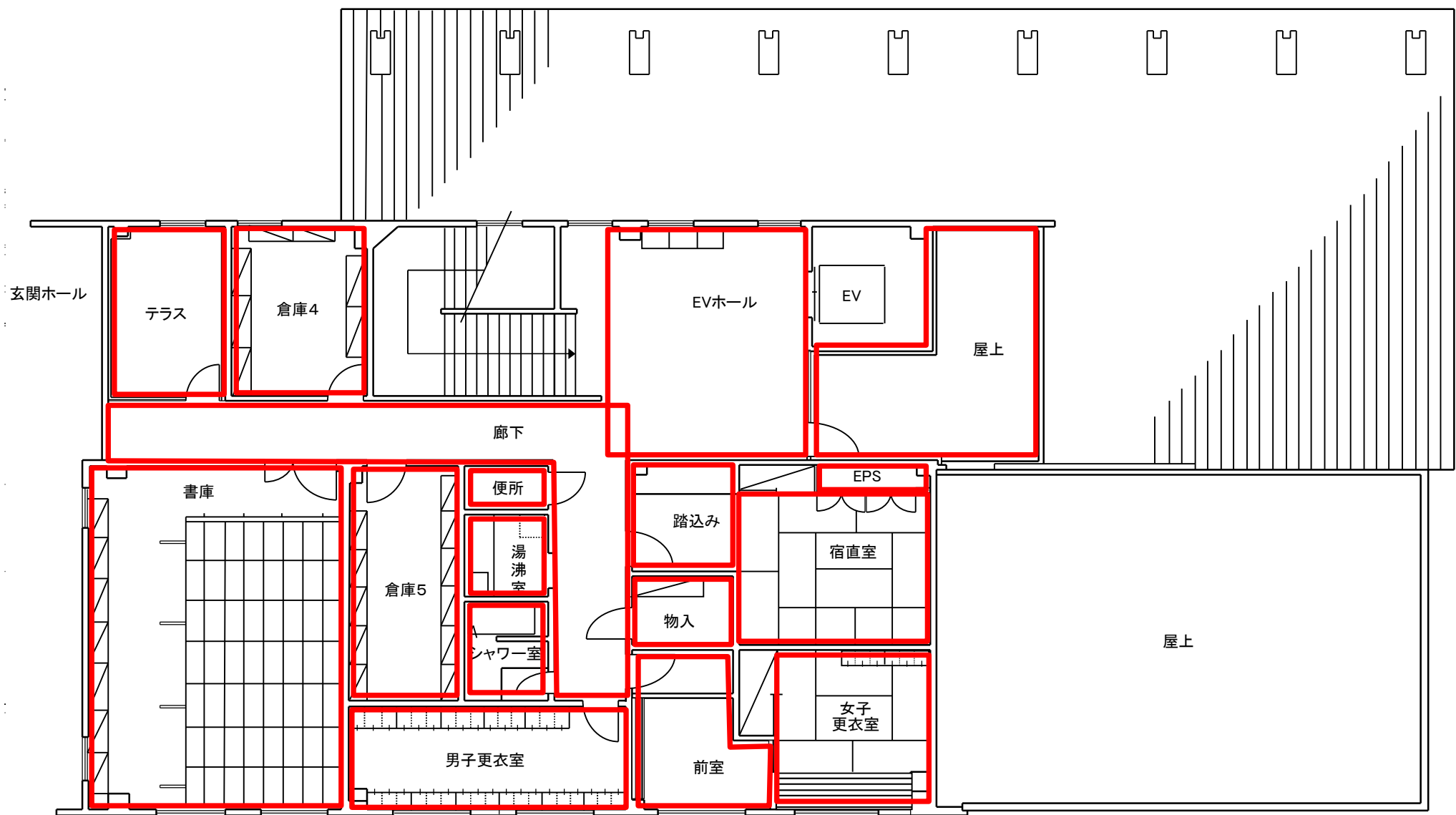
松本労働基準監督署 3階平面図
