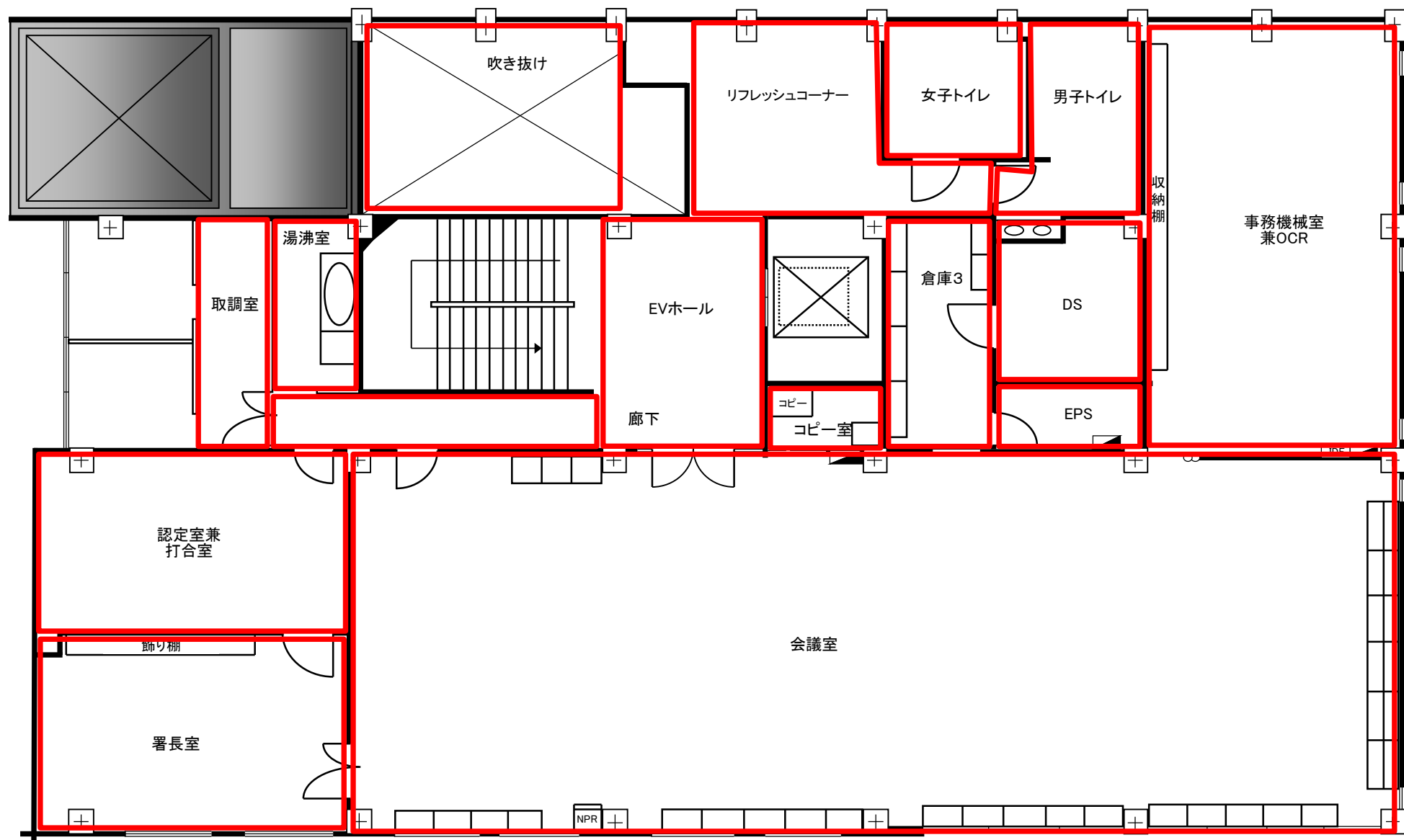
松本労働基準監督署 2階平面図
