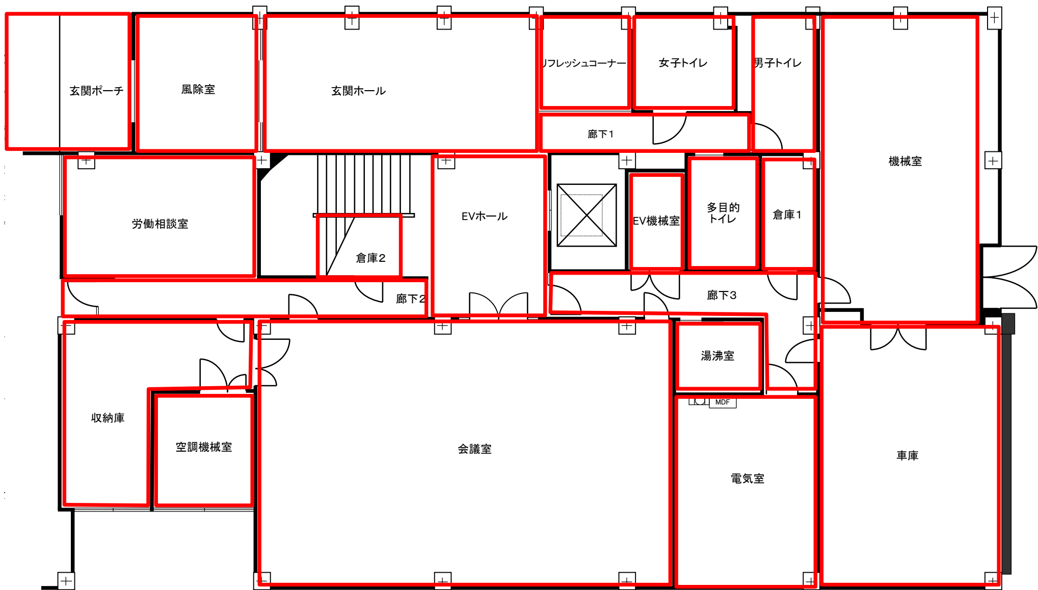
松本労働基準監督署 1階平面図
