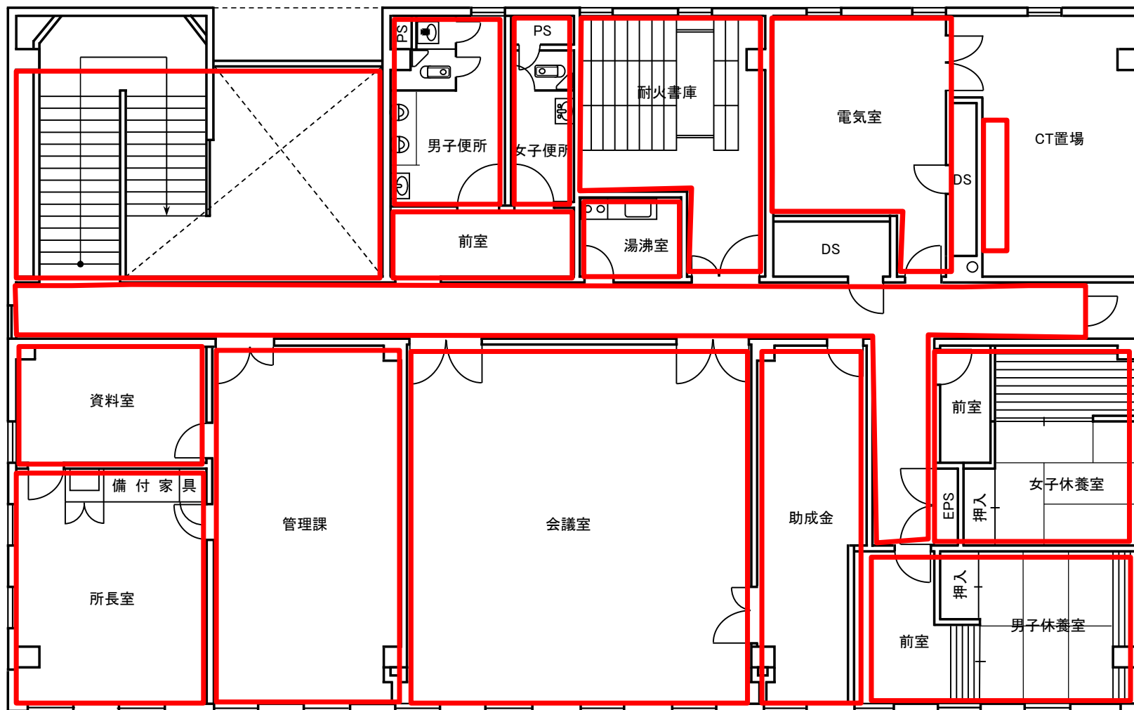
佐久公共職業安定所 2階平面図
