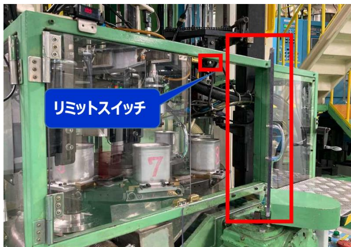
機械装置は、本質安全化を推進しています。 安全装置の動作確認も行いました。
