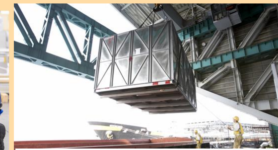
完成したスチールケースと130トンの貨物が吊れる天井クレーン
