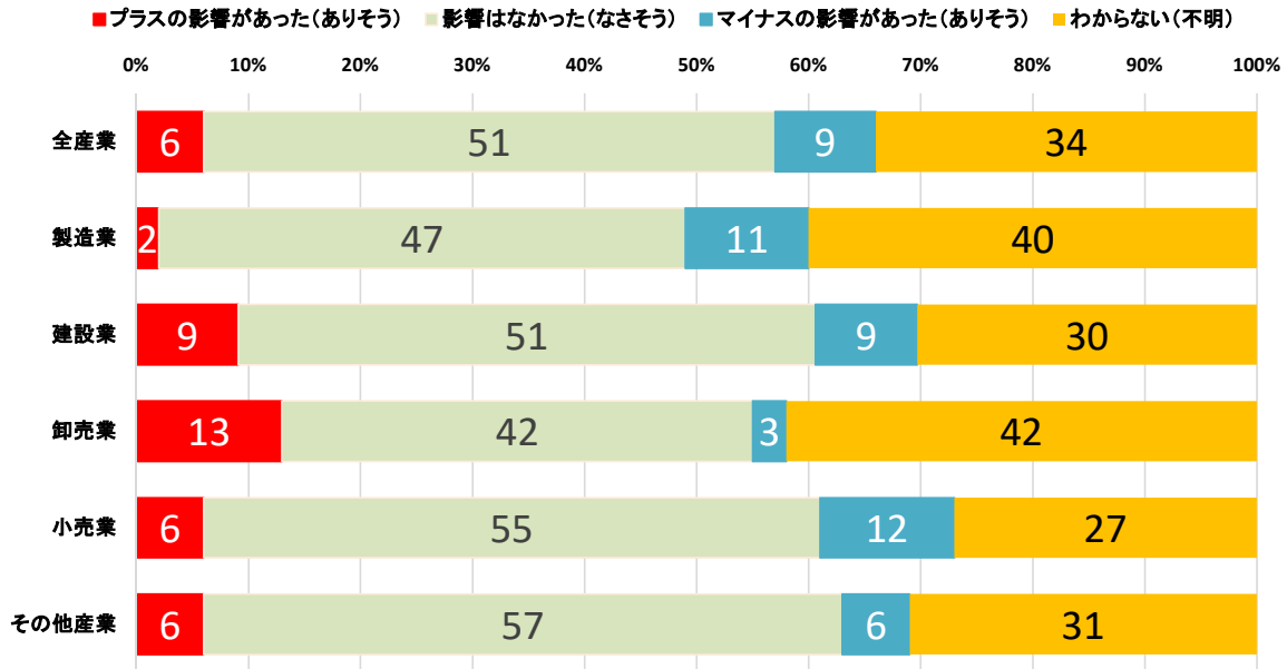
図表13-1 TSMCの熊本県進出による自社への影響
