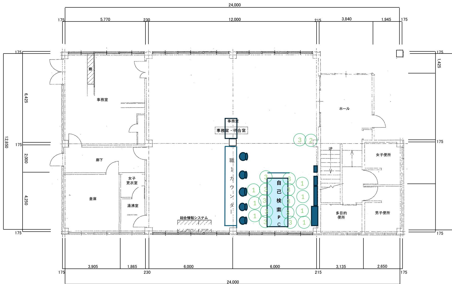
1階平面図
