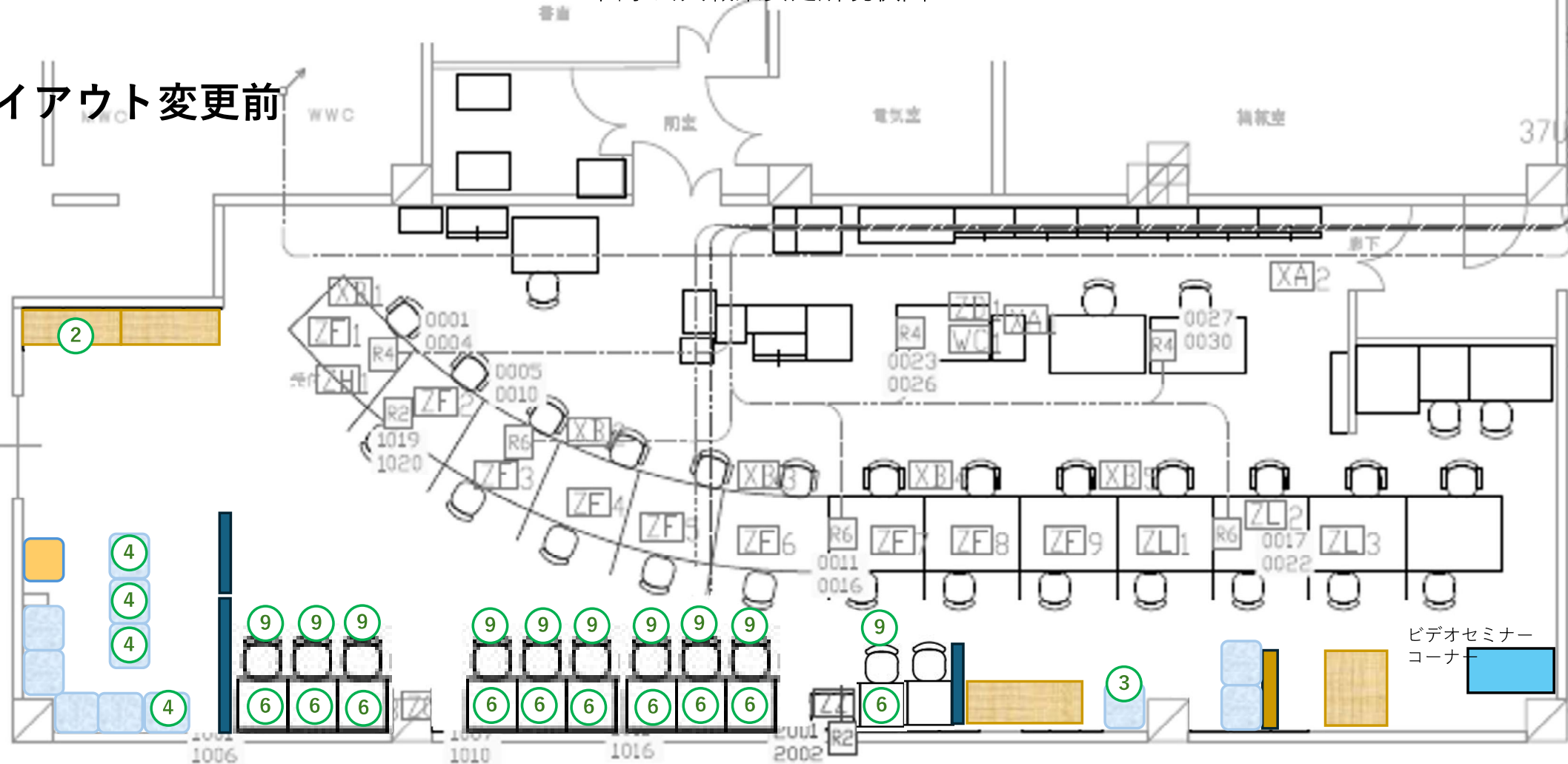
出水公共職業安定所現状図
