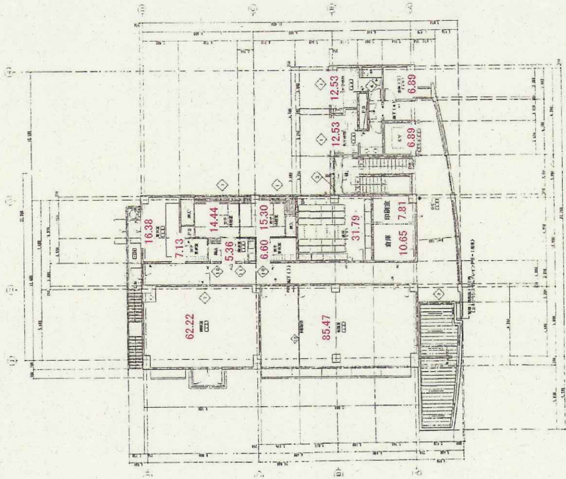
2 階平面図 (川内公共職業安定所富之島出張所)
