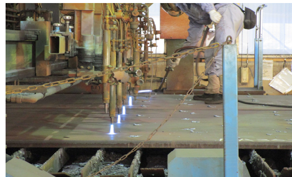
■炎を再点火しています（炎を当てて鋼材を切断）
