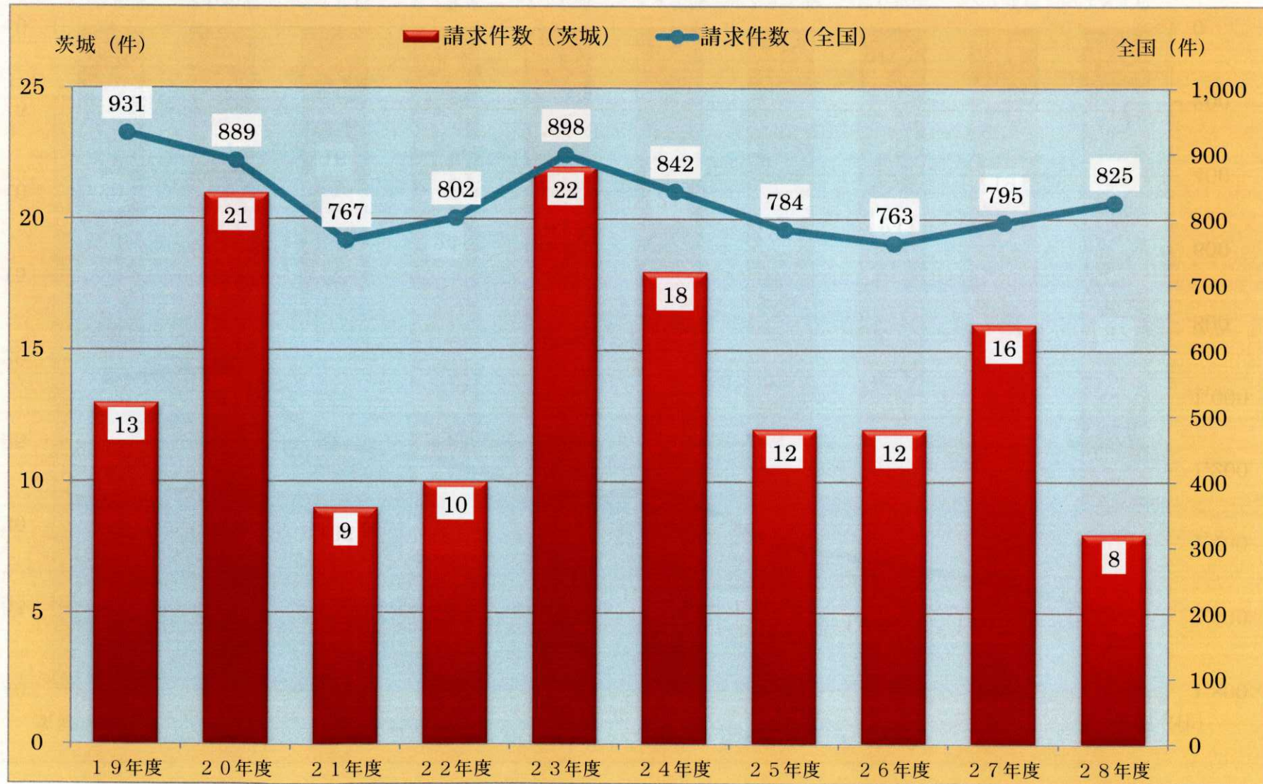
全国と茨城労働局内における脳・心臓疾患の労災請求件数の推移（平成 19～28 年度）
