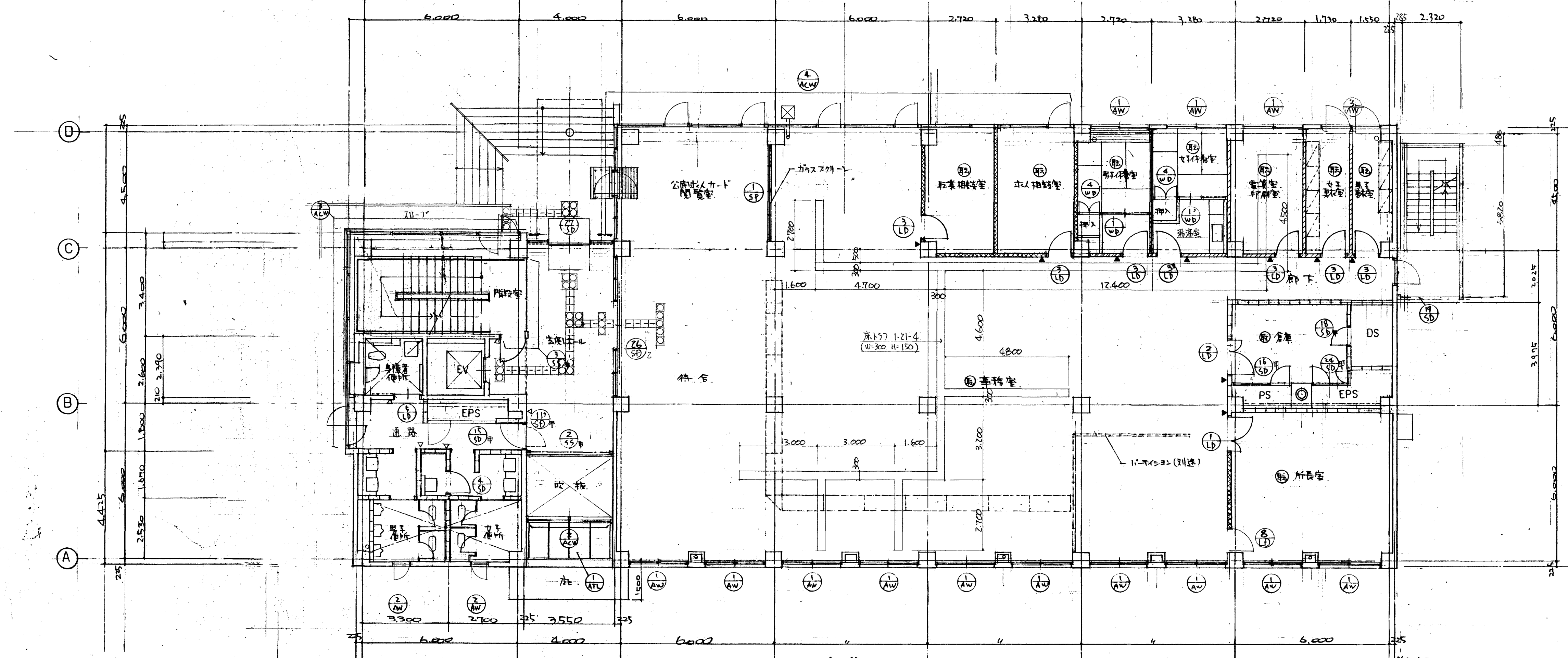
2階平面図 1/100
