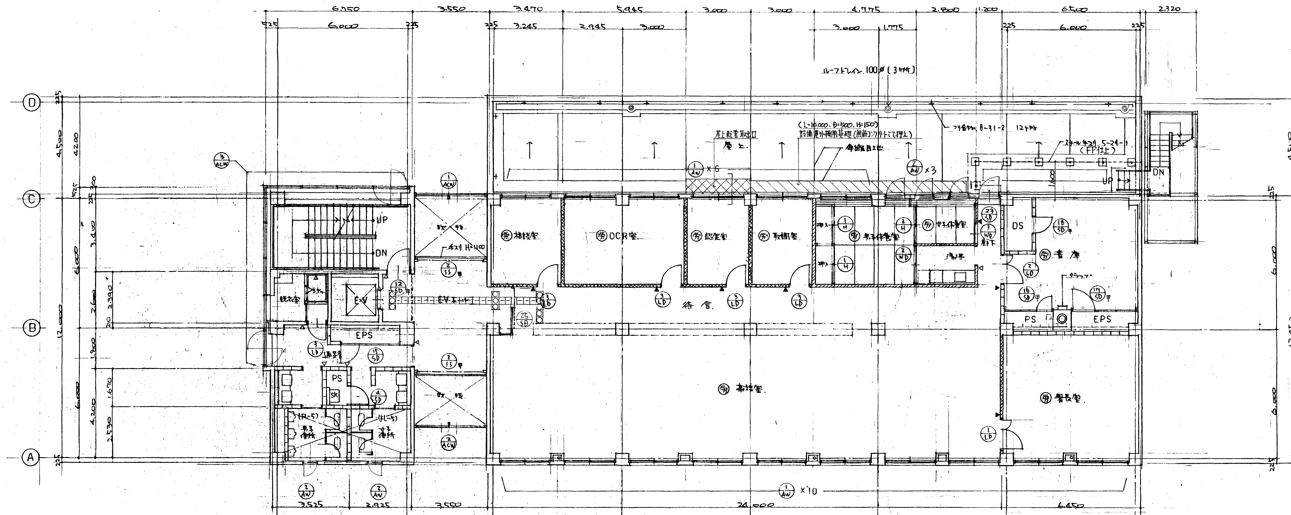
4階平面図 1/100
