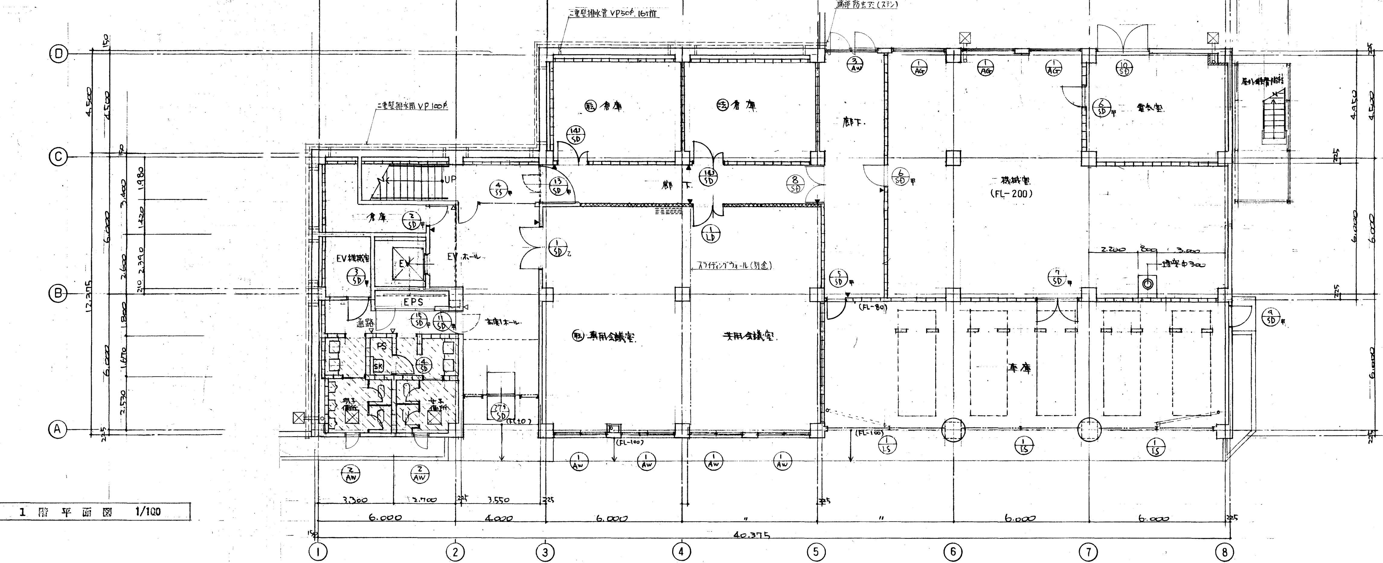
1階平面図 1/100
