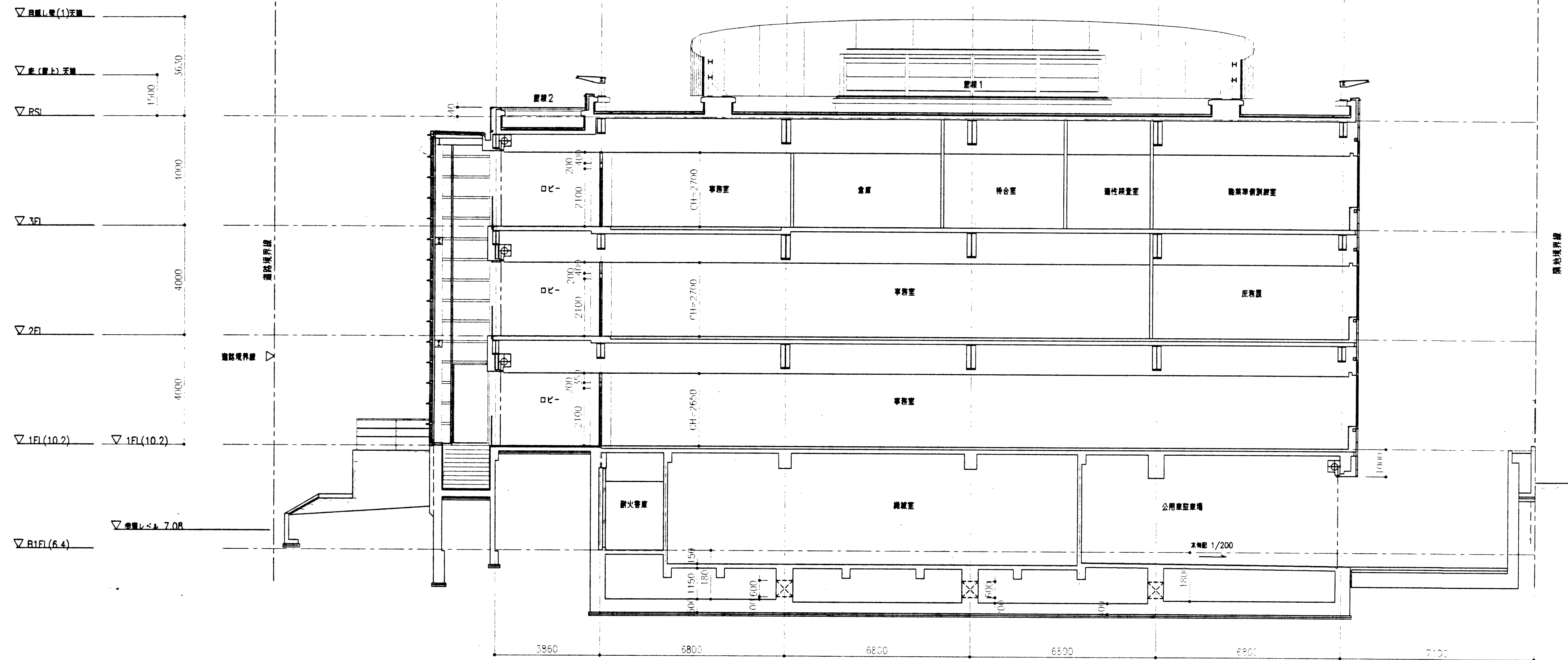
断面図 1
