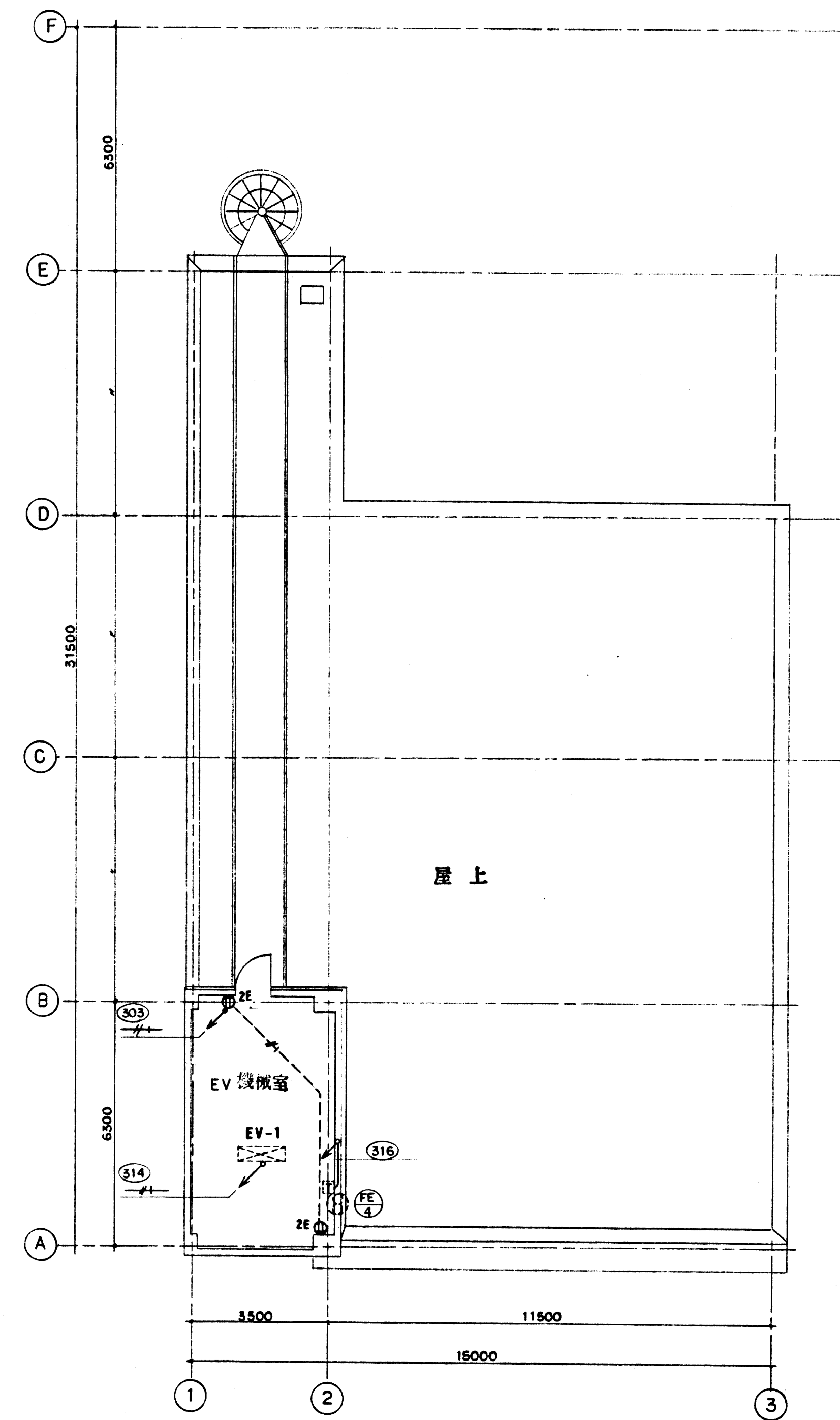
屋階平面図
