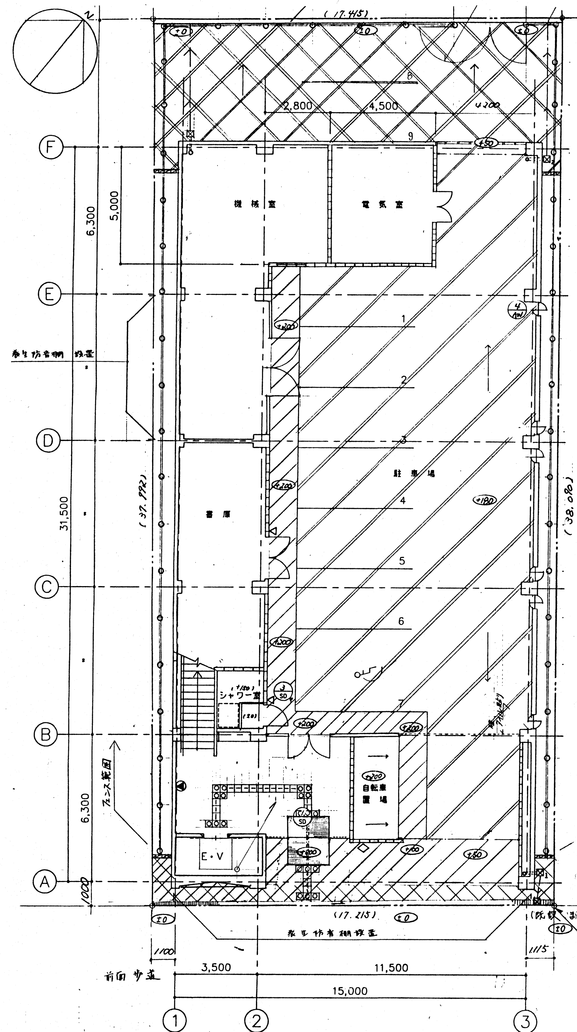
1 階 平 面 図 S : 1/100
