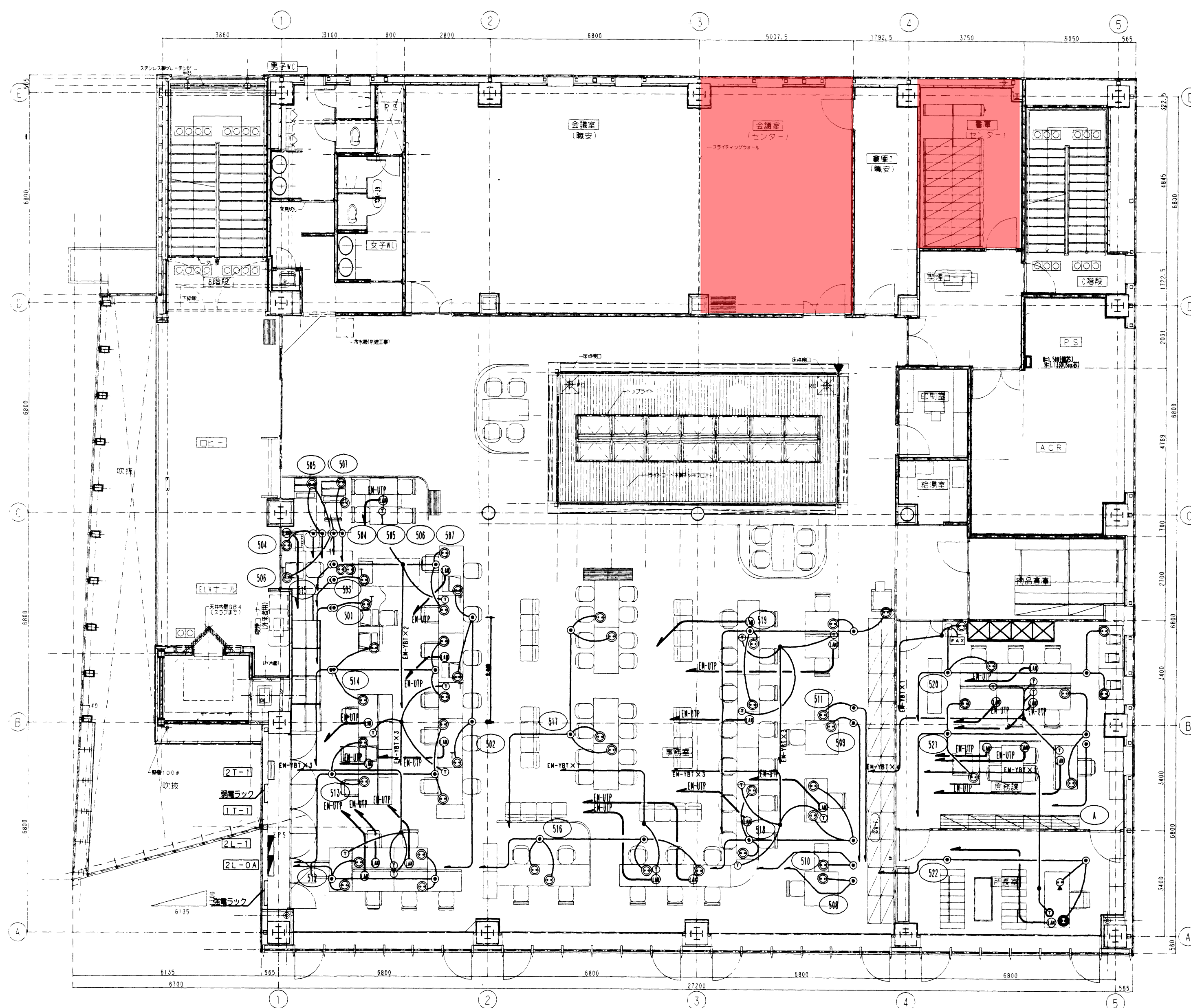
2階平面図
