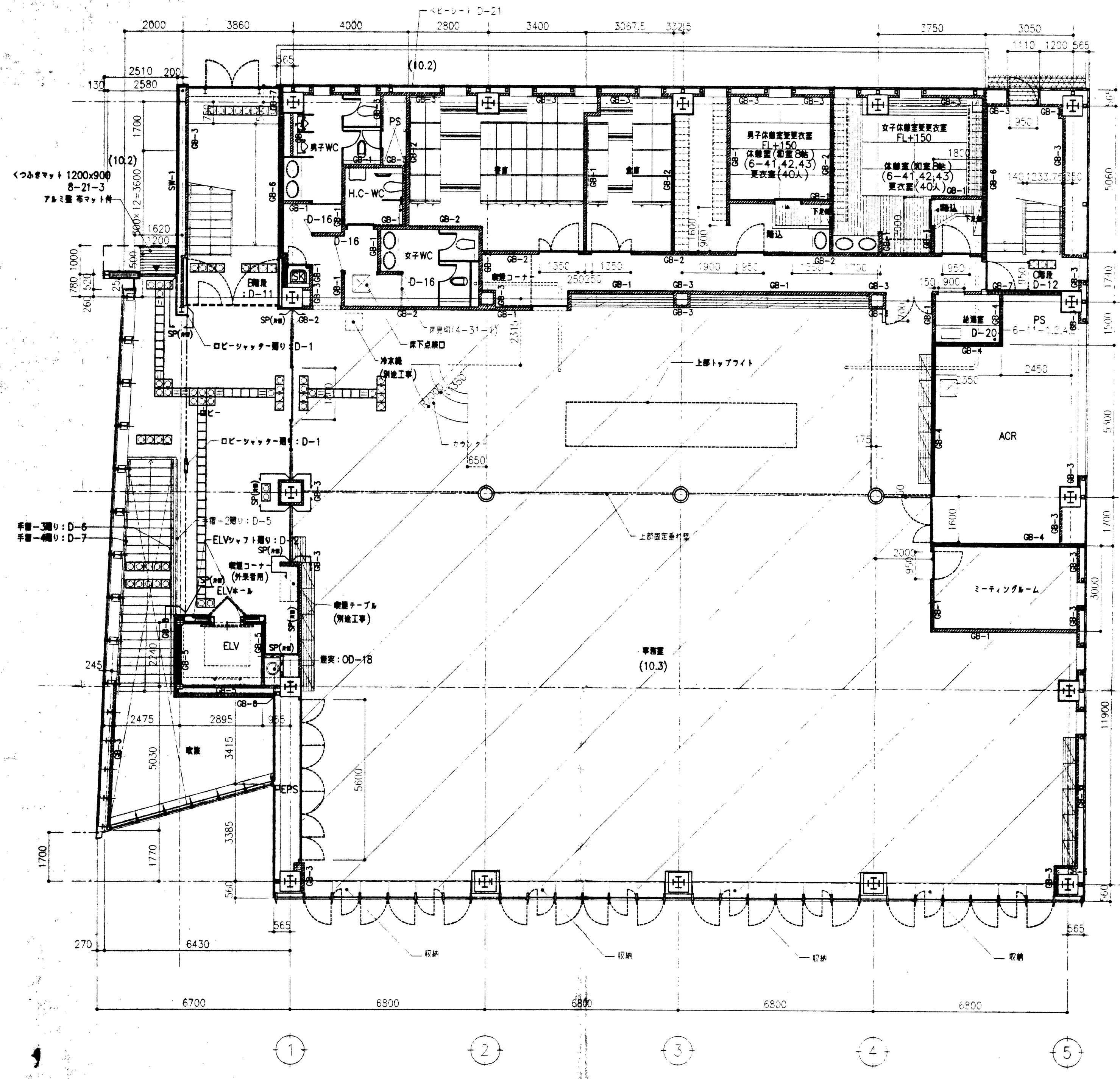
1階平面図
