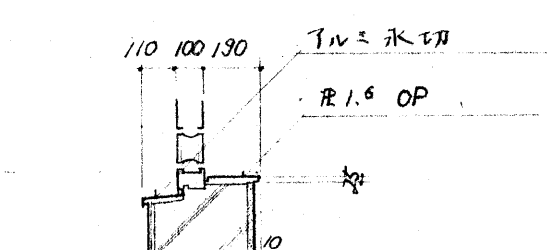
① 部 詳細図 S. 1: 30
