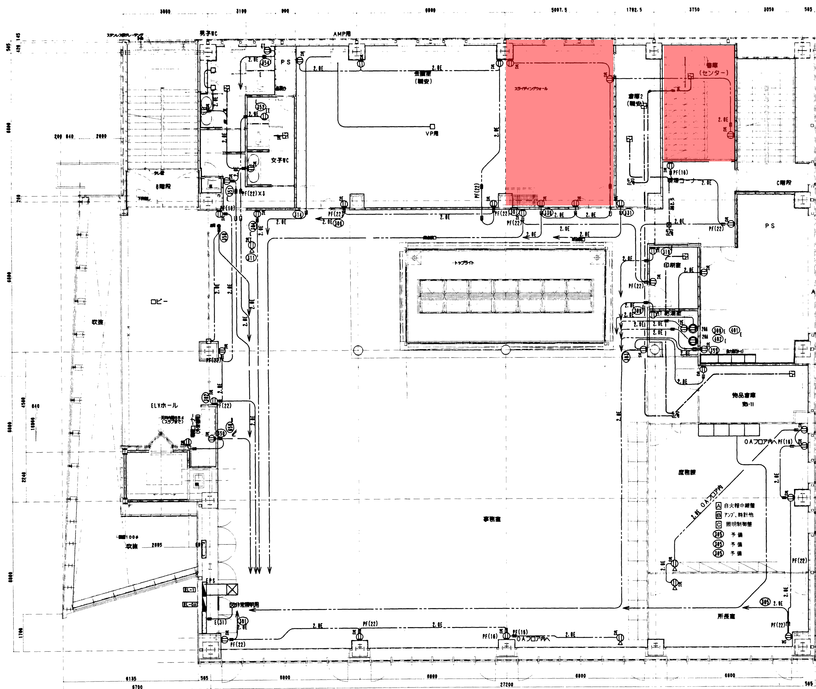
2階平面図
