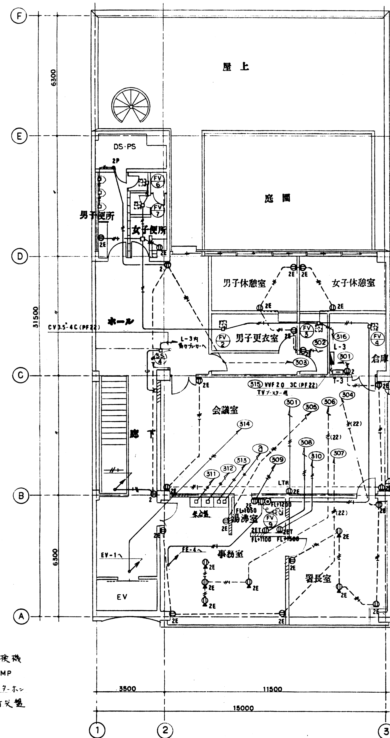
3F 平面図
