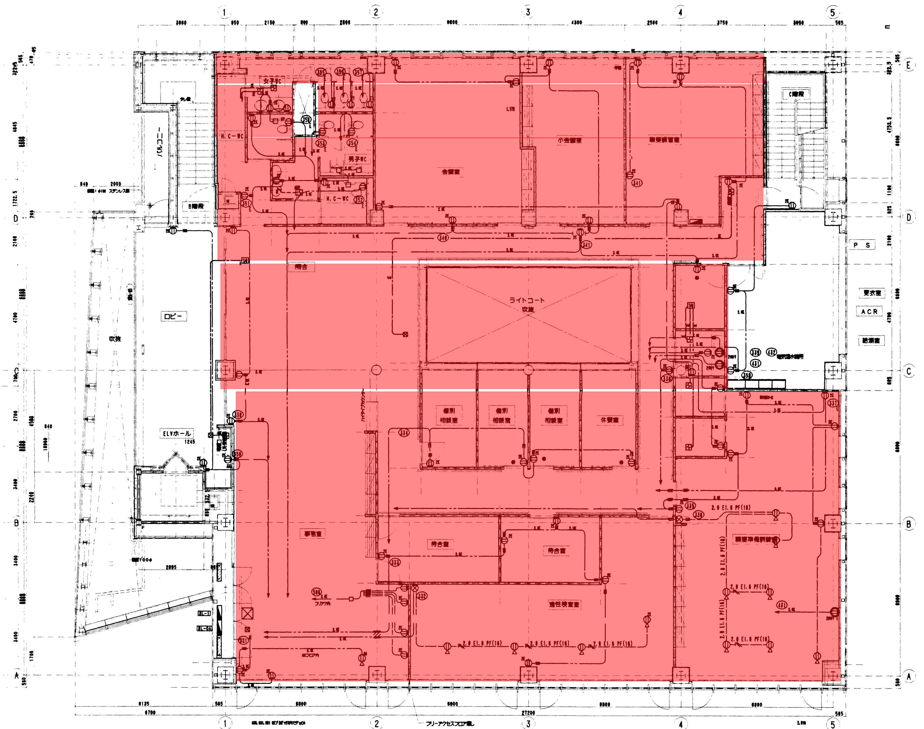
3階平面図
