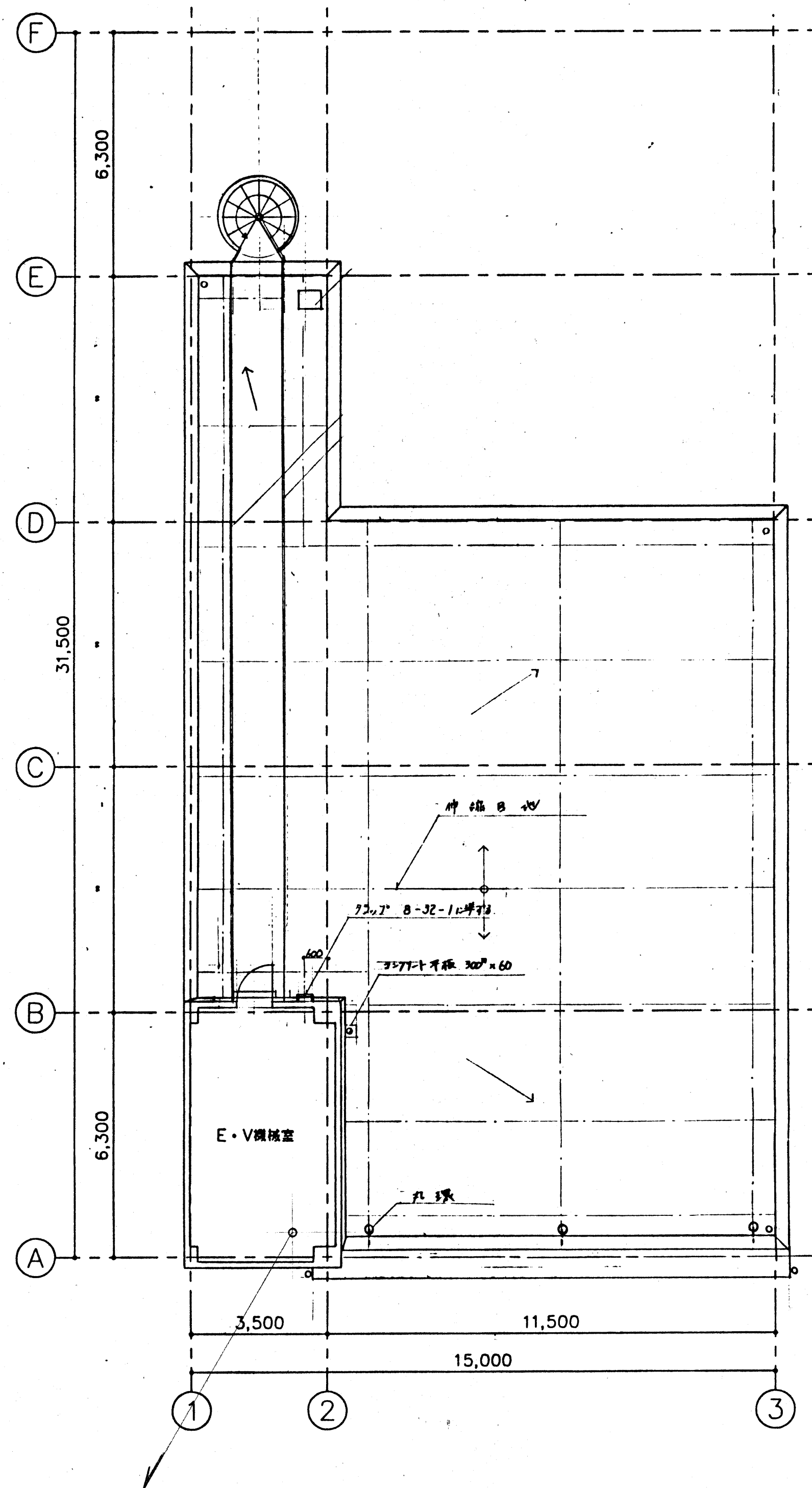
屋 階 平 面 図 S:1/100
