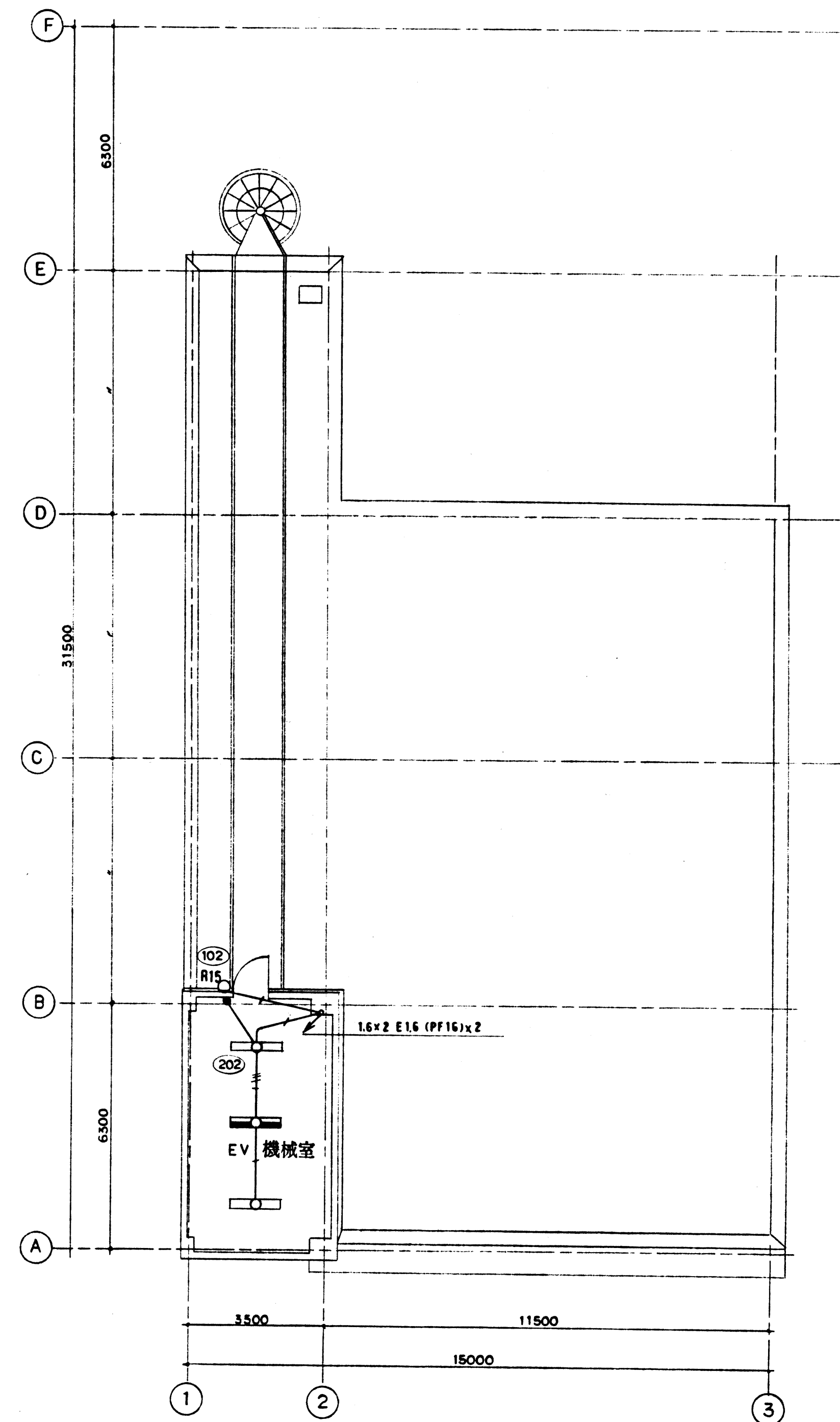
屋階平面図
