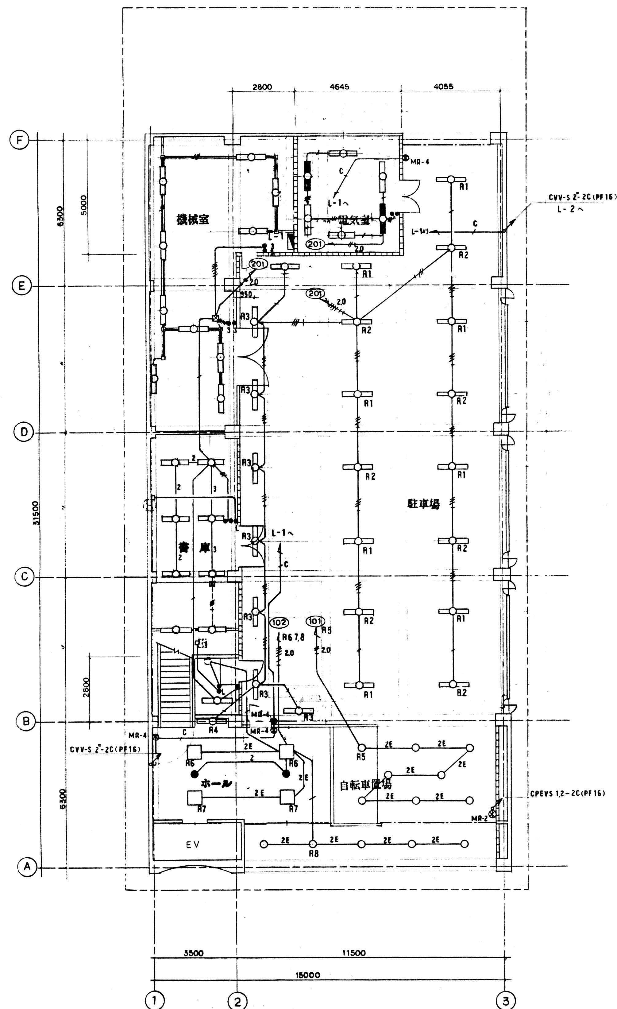
1 F 平面図
