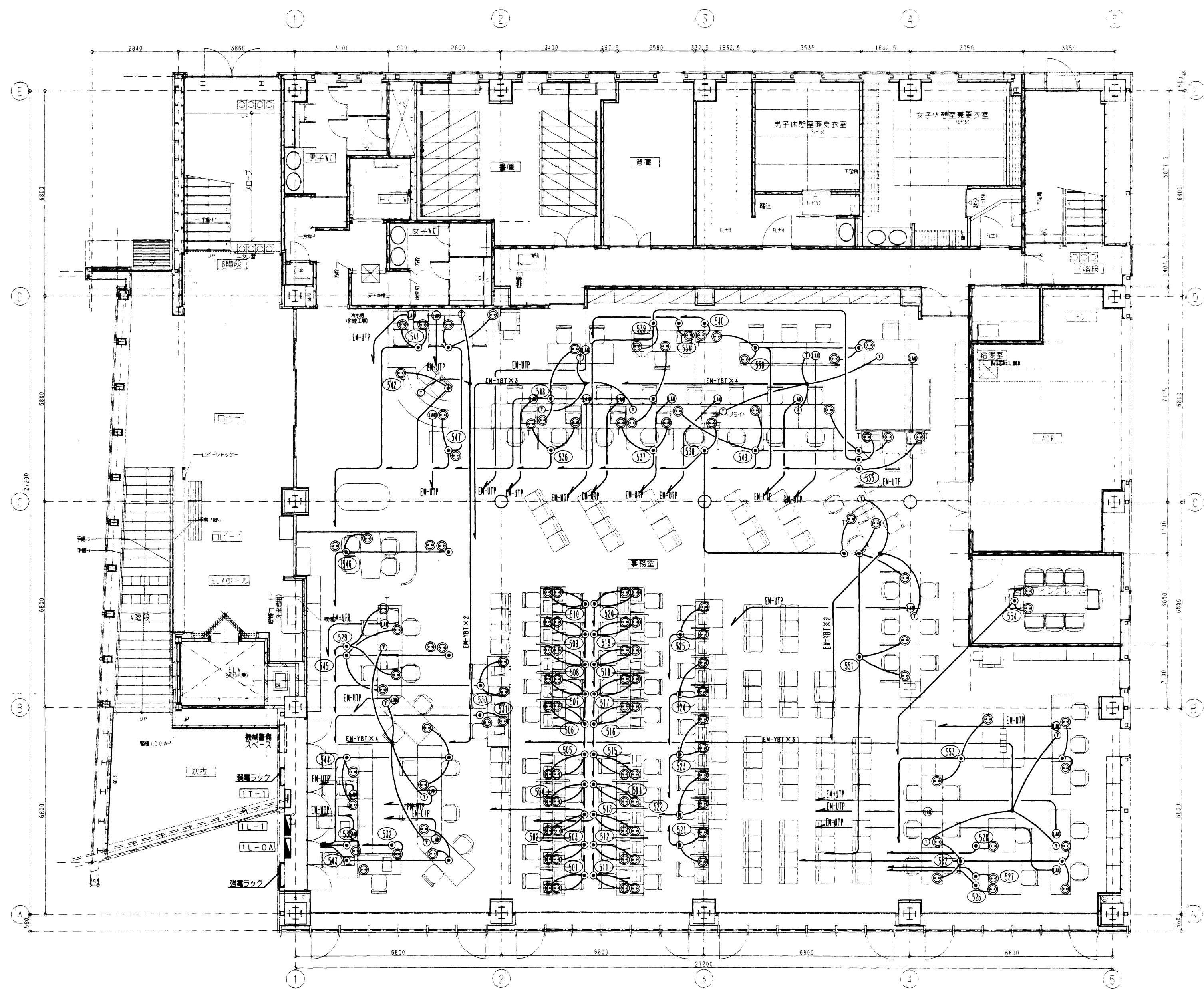
1階平面図
