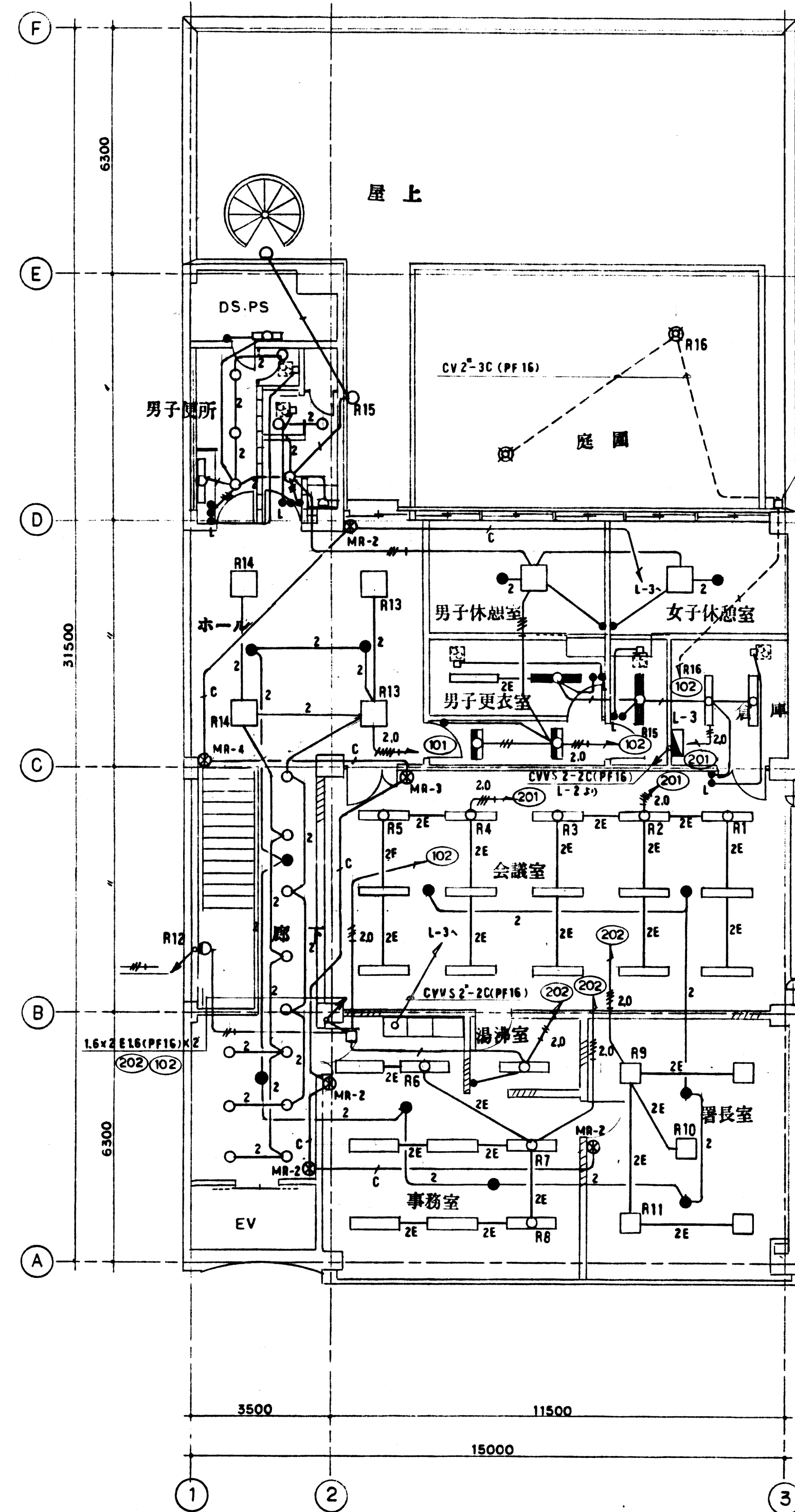
3 F 平面図
