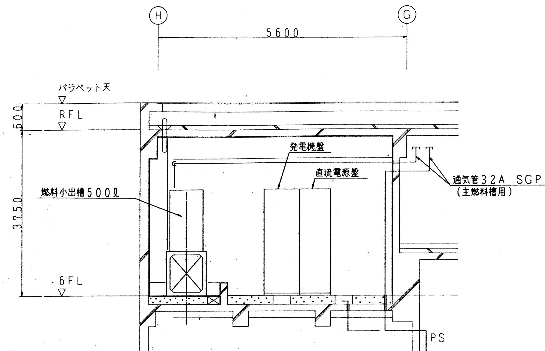
B-B断面図 S=1/50
