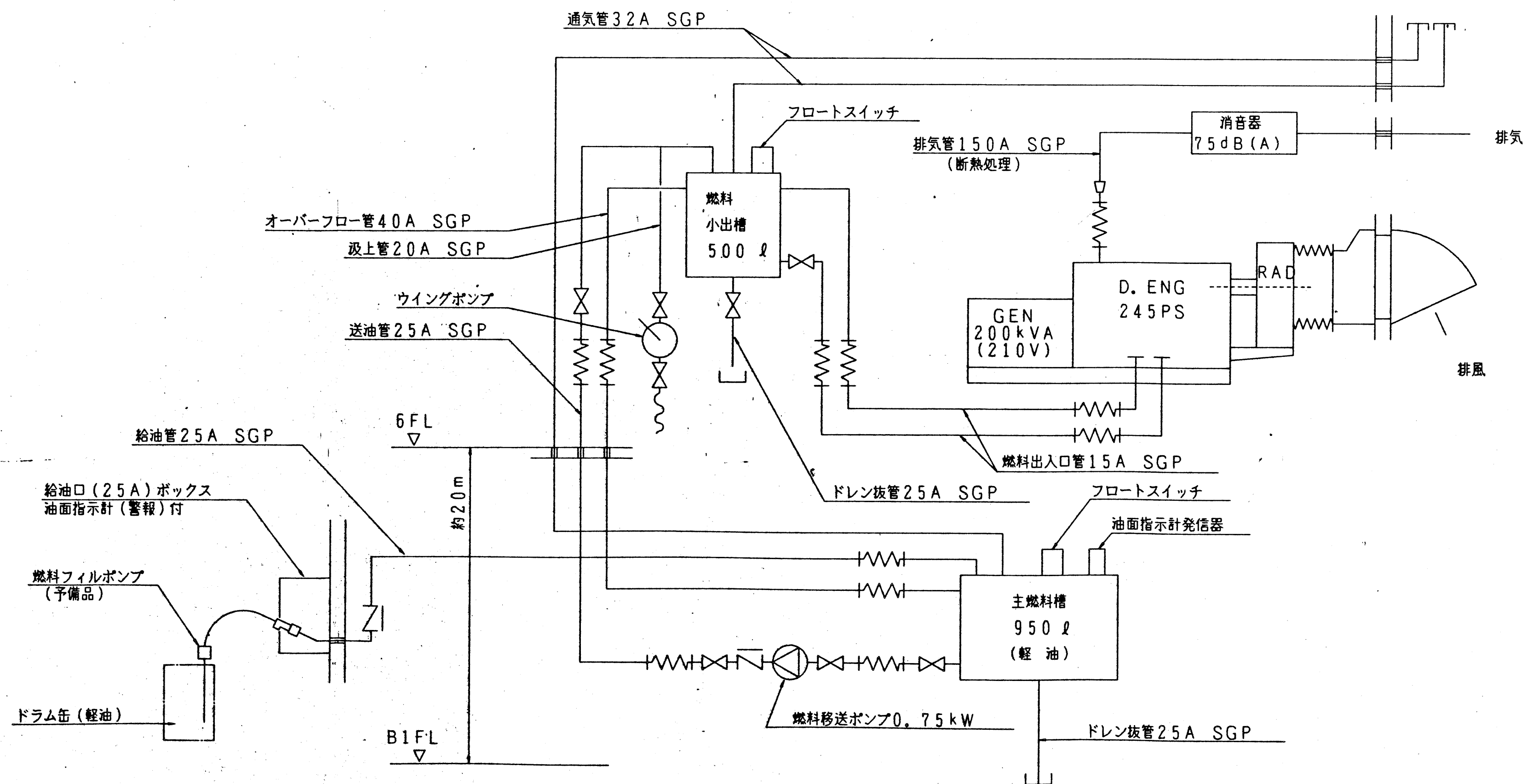
配管系統図
