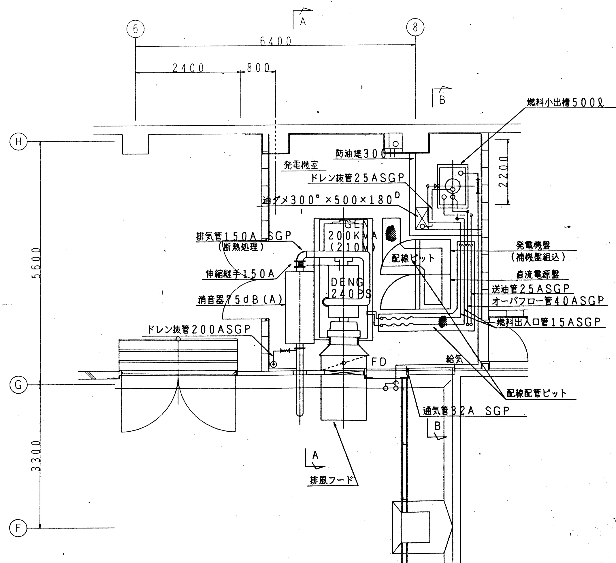
6F発電機室平面図 S=1/50
