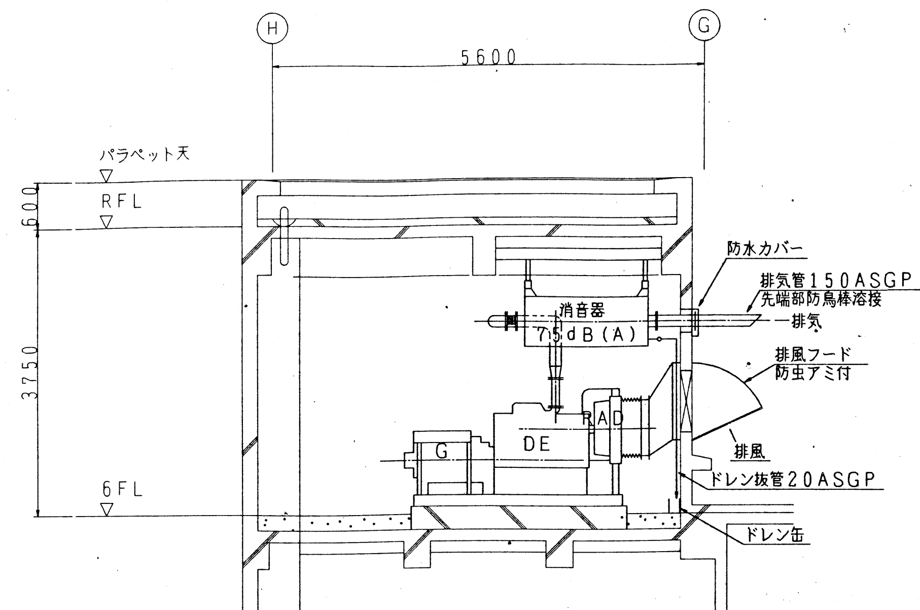
A-A断面図 S=1/50
