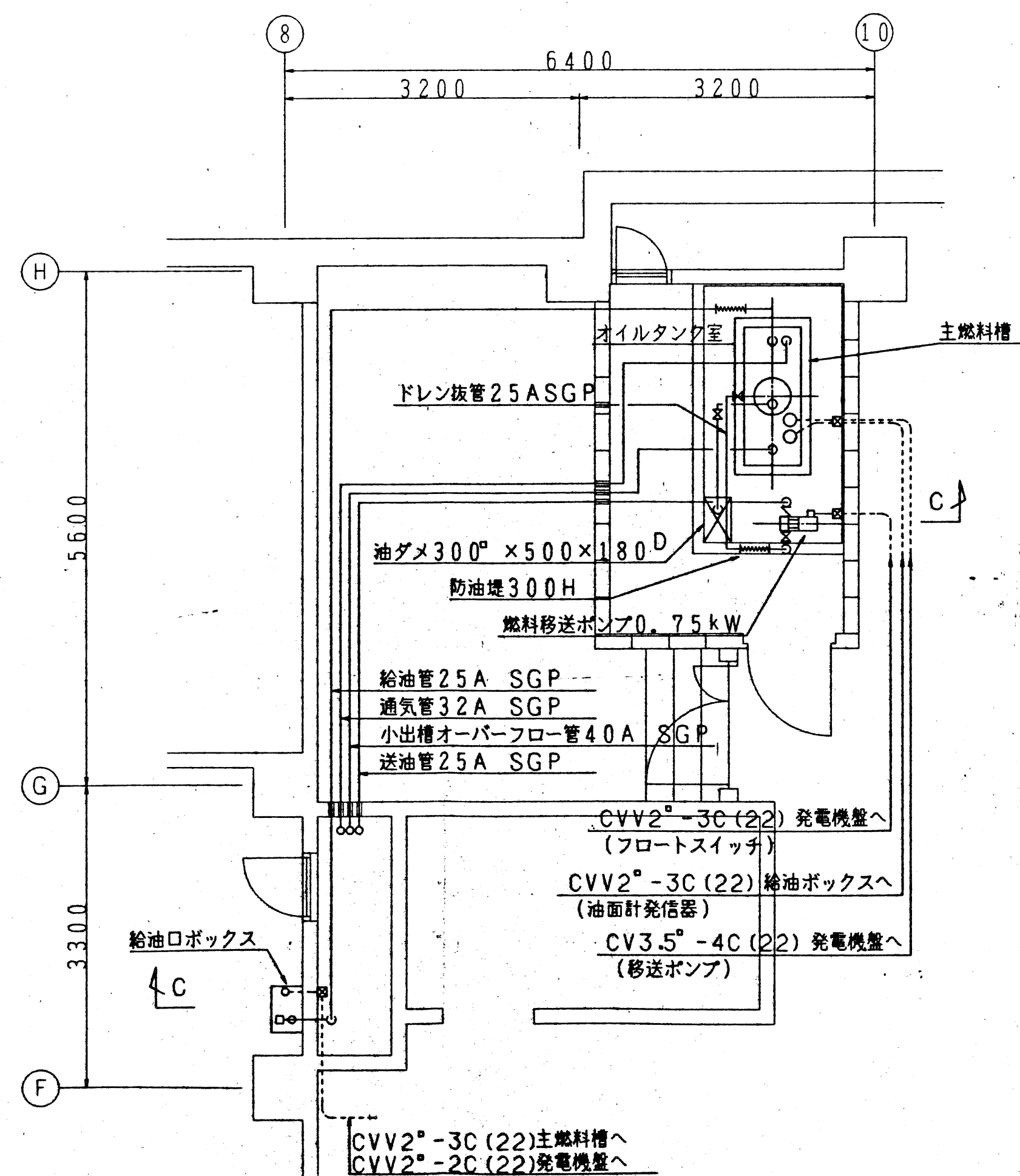
B1Fオイルタンク室平面図 S=1/50
