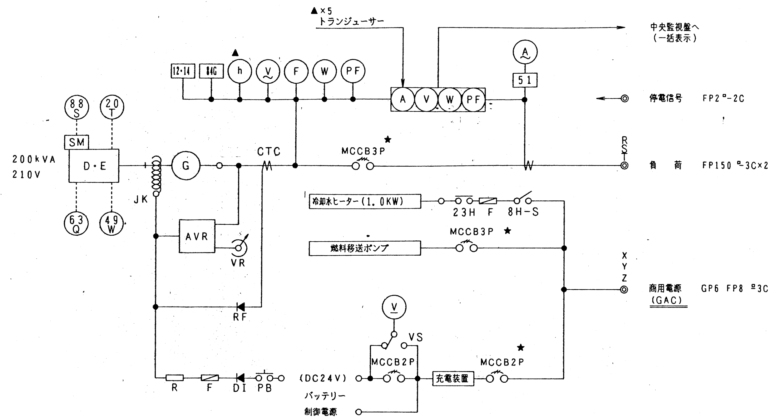
單線結線図
