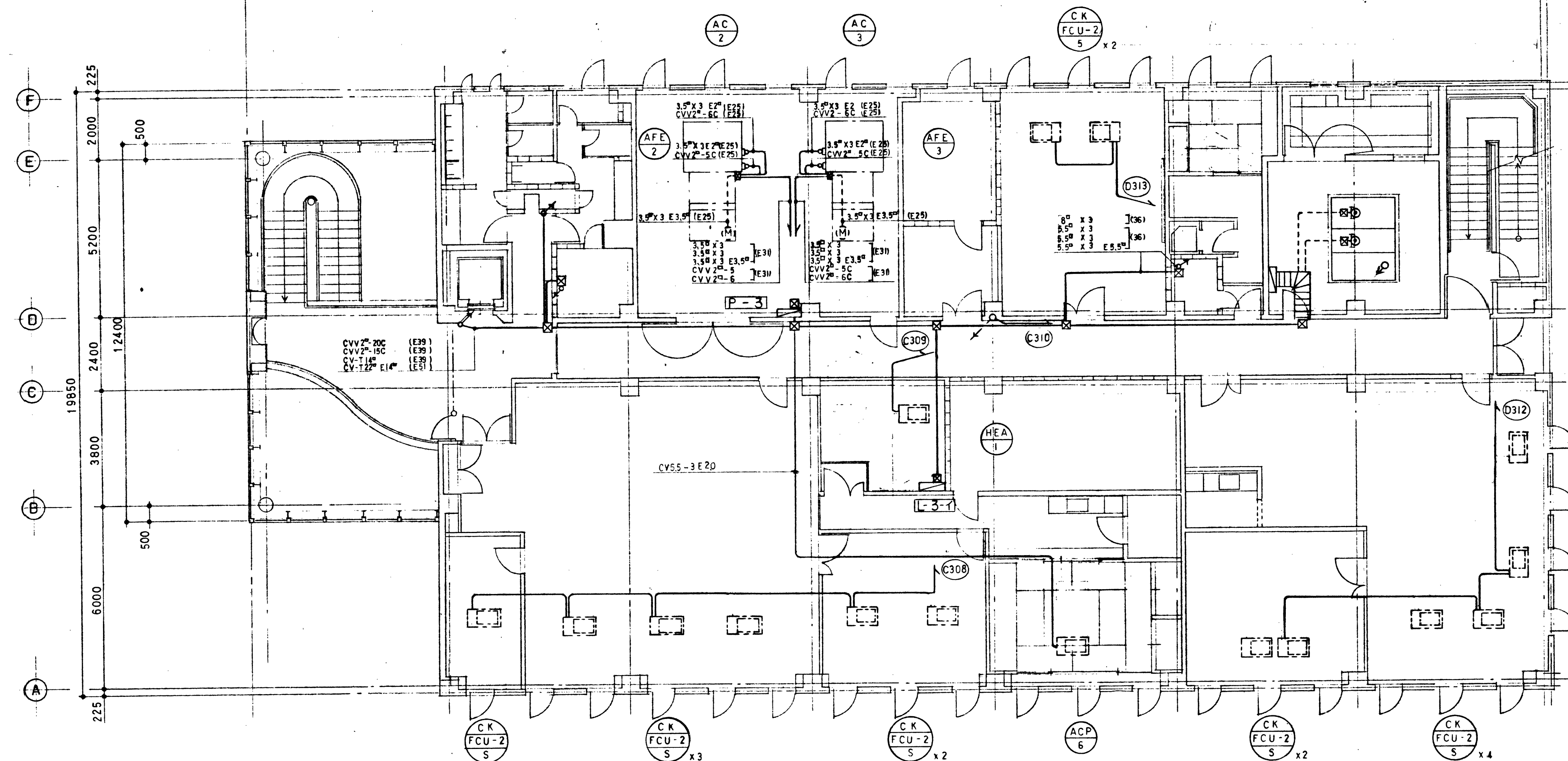
3階平面図 1/100
