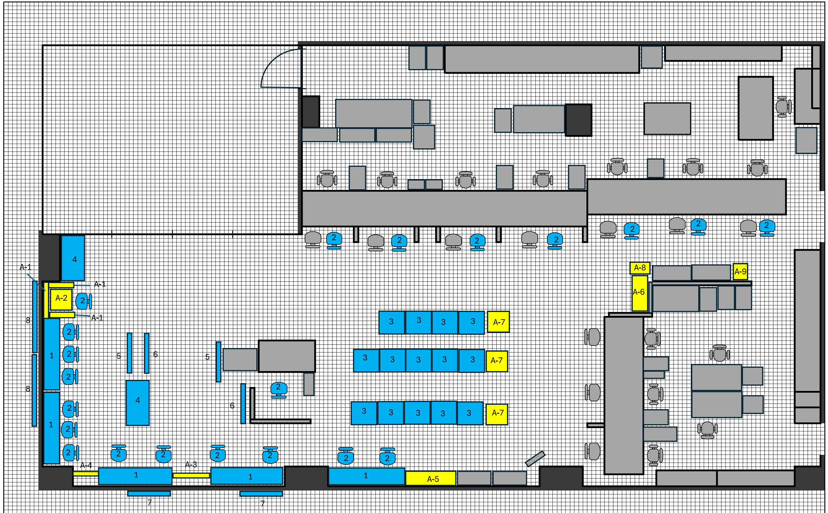
【相生所】レイアウト図（変更後）
