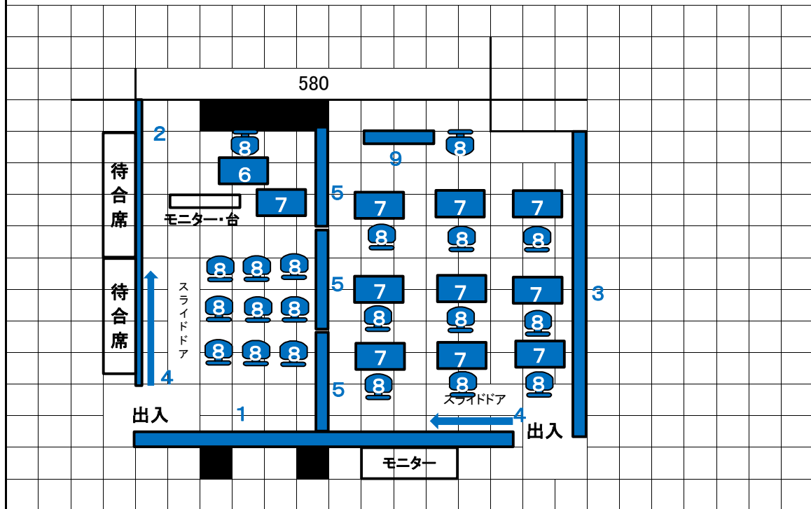
【姫路所】レイアウト図(変更後:東館1階_セミナースペース)
