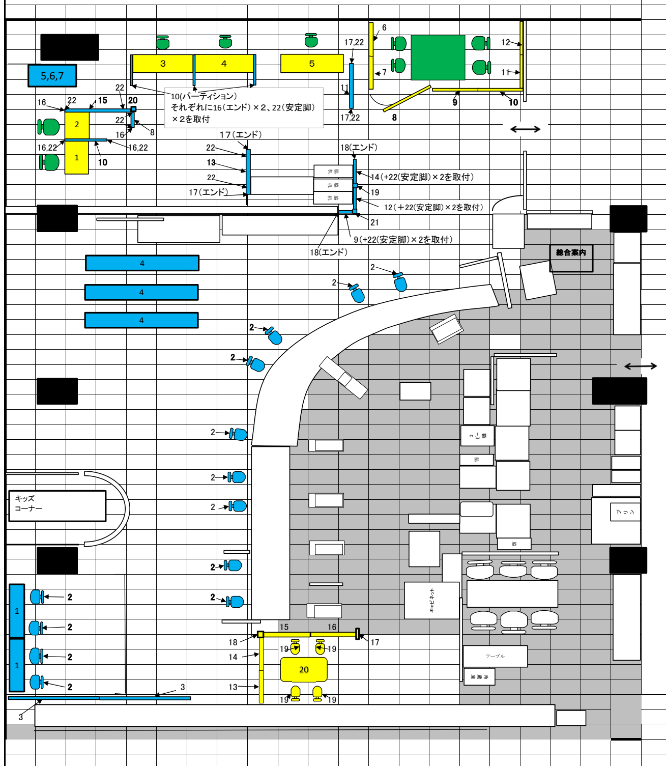
豊岡公共職業安定所 1F レイアウト図（変更後）
