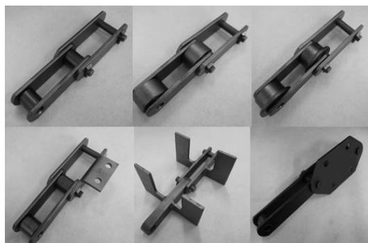
当社製作品(コンベヤチェーン)
