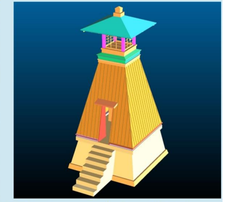
地上レーザ計測結果からのモデリング事例
