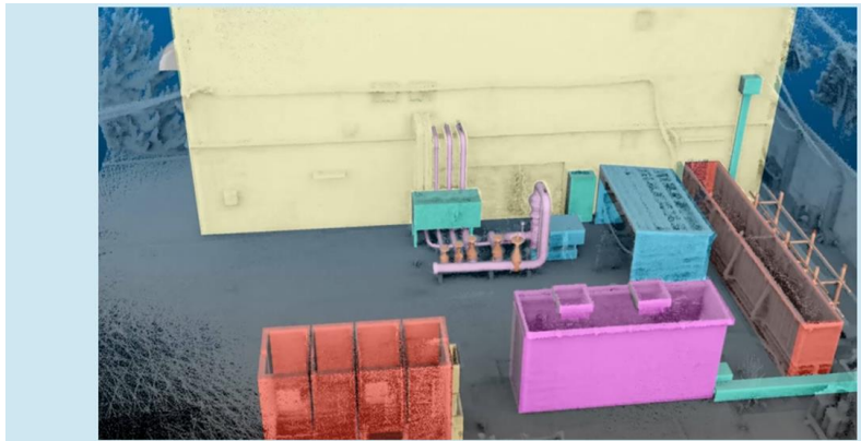
ハンディ型レーザスキャナ計測結果からのモデリング事例
