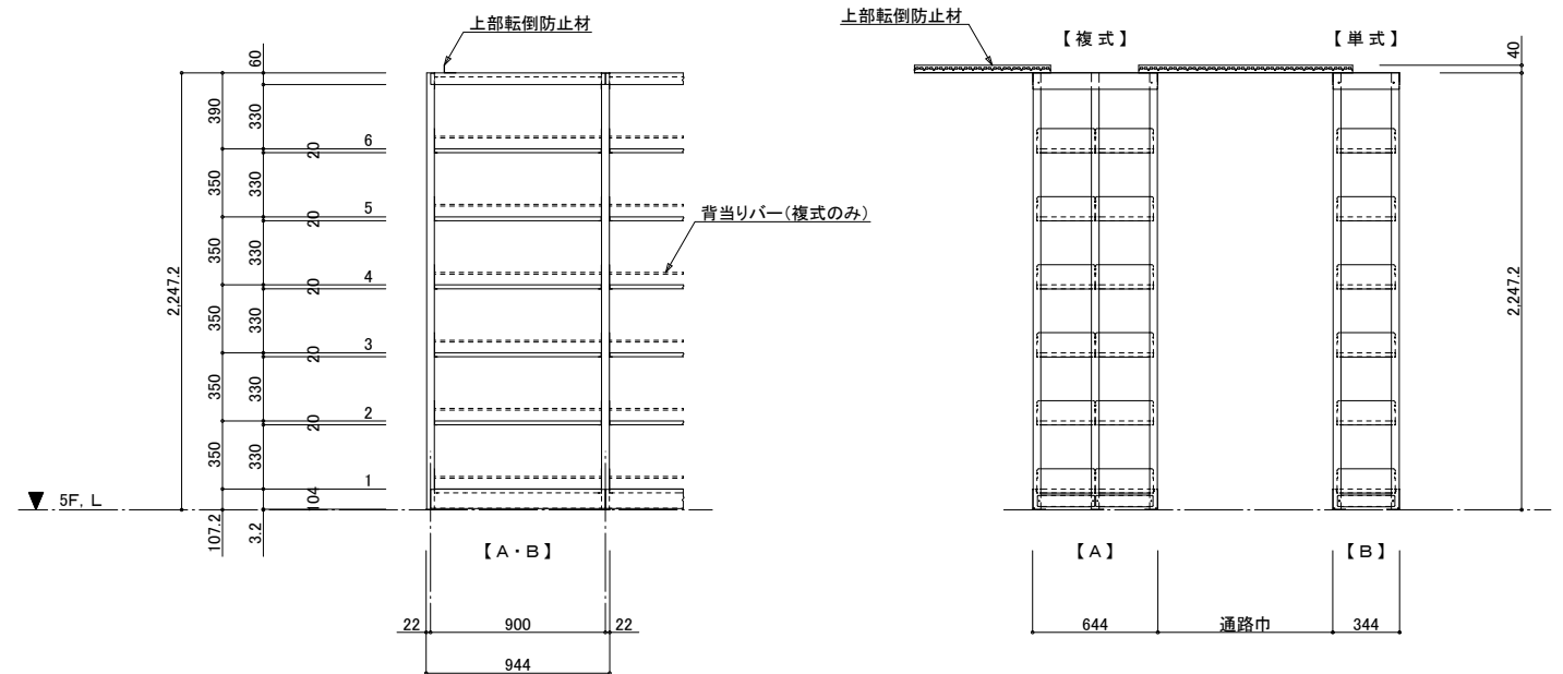
複柱書架 姿図【A・B】 S = 1 : 30
