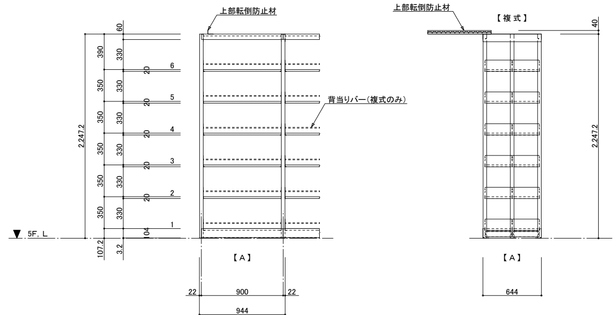
複柱書架 姿図【A】 S = 1 : 30
