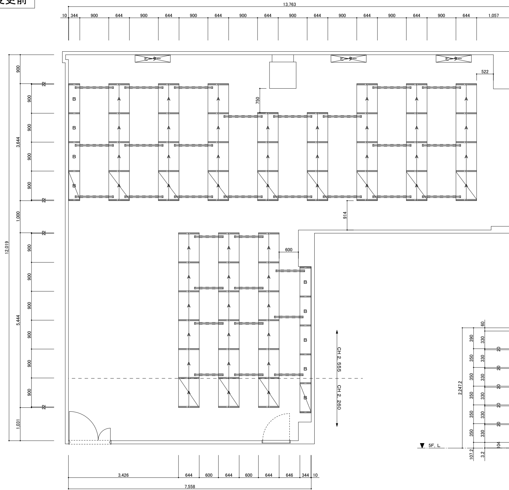
5階【書庫室】配置図 S = 1 : 50
