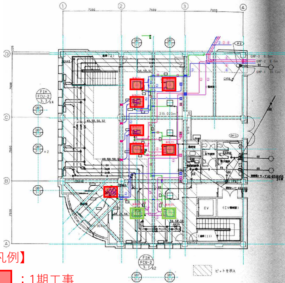
1階空調配管平面図 S=1/100
