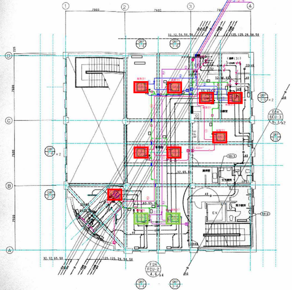
2階空調配管平面図 S=1/100
