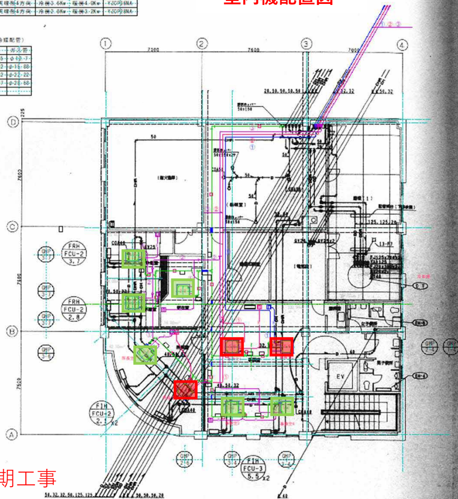
3階空調配管平面図 S=1/100
