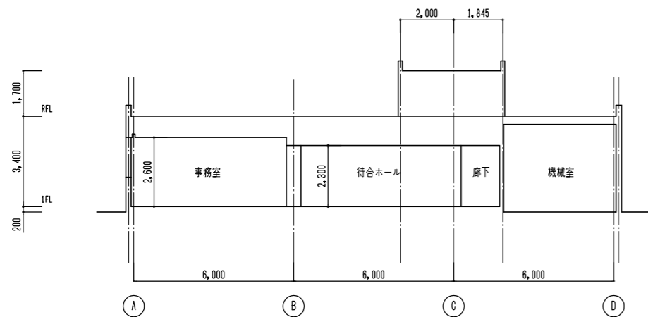
断面図 S=1/100
