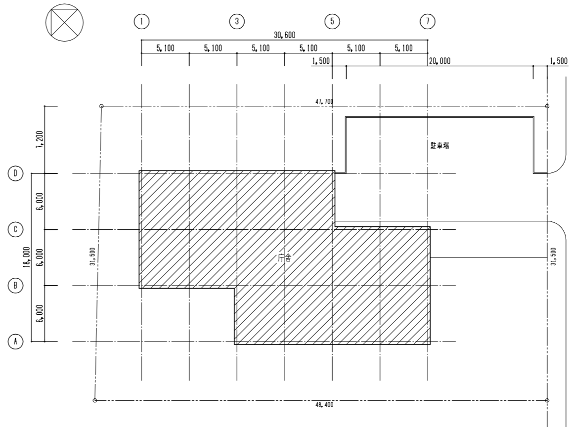
配置図 S=1/200
