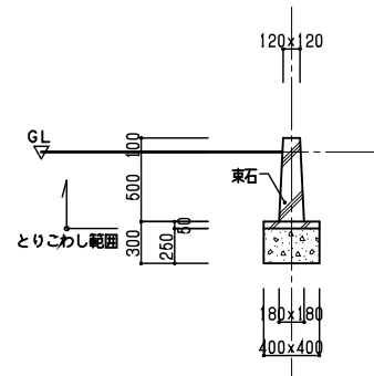
東石 S=1/30
