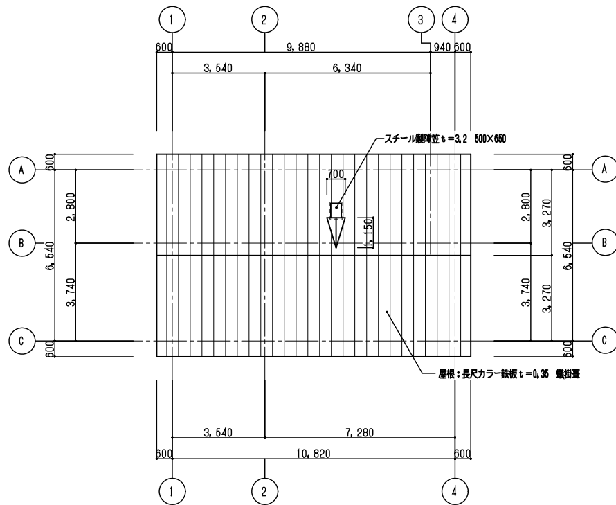
屋根伏図 S=1/100
