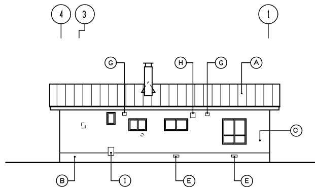
北立面図 S=1/100
