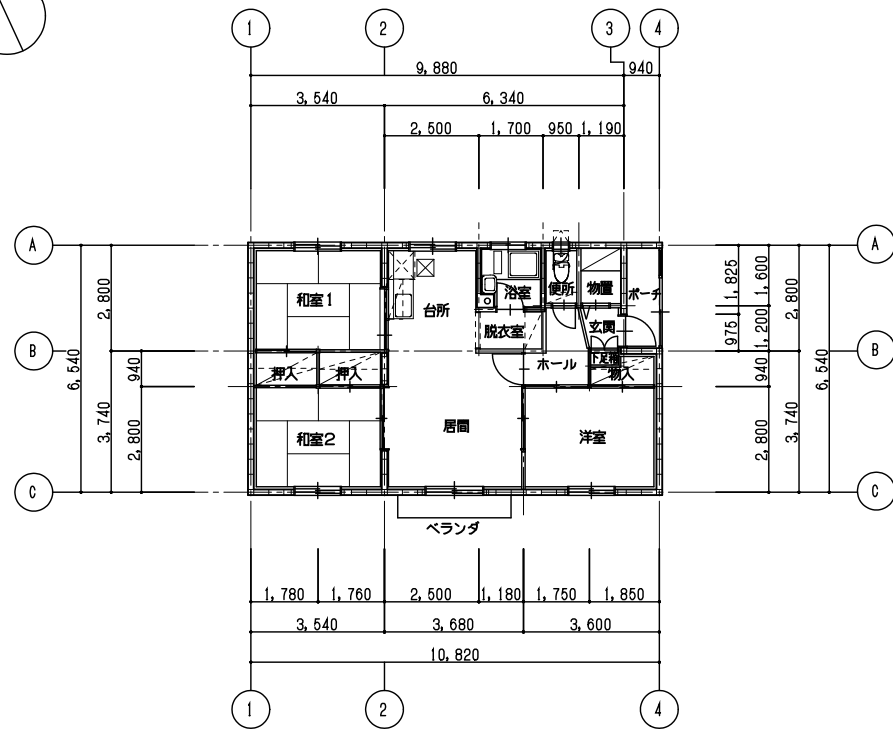
平面図 S=1/100
