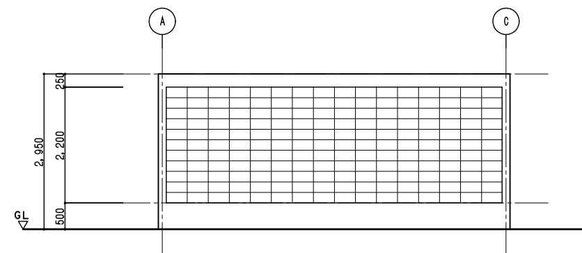
1通ブロック割図 S=1/50
