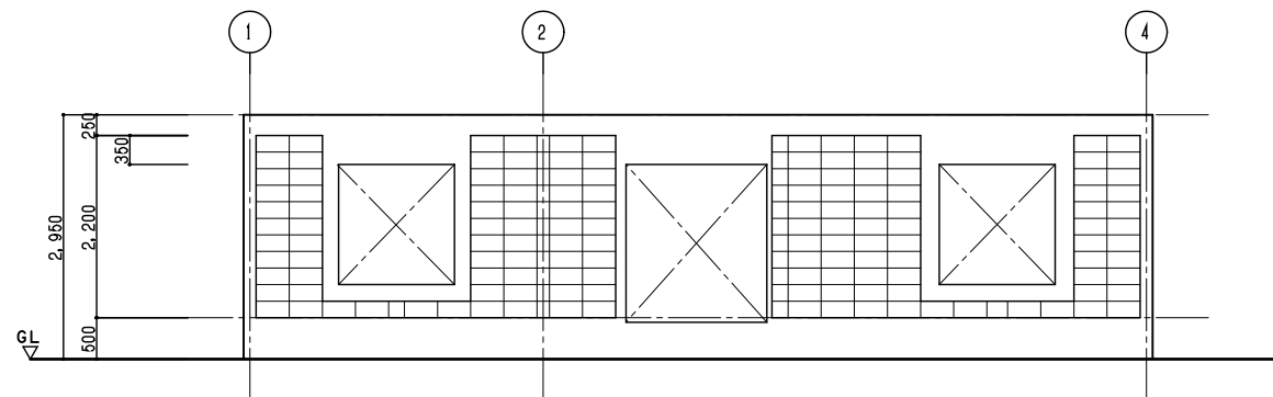
C通ブロック割図 S=1/50
