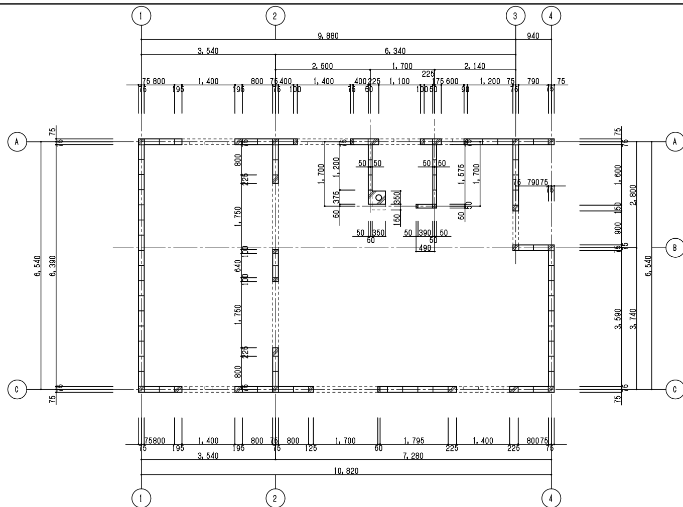
ブロック割平面図 S=1/50
