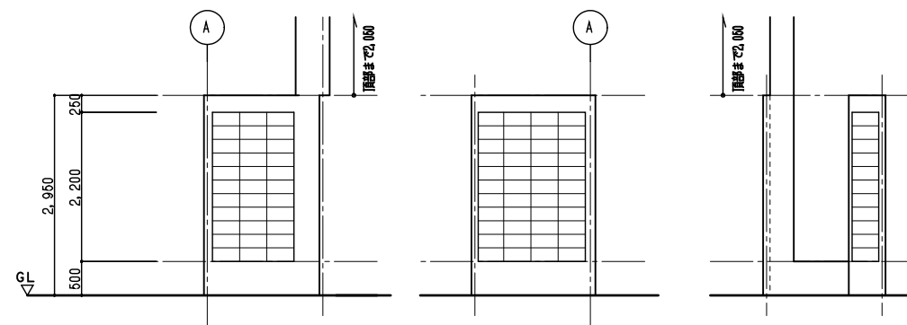
浴室廻りブロック割図 S=1/50
