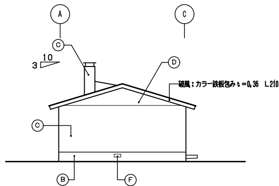
西立面図 S=1/100
