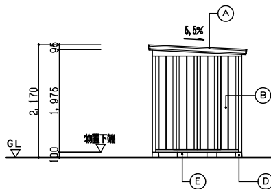
南立面図 S=1/50
