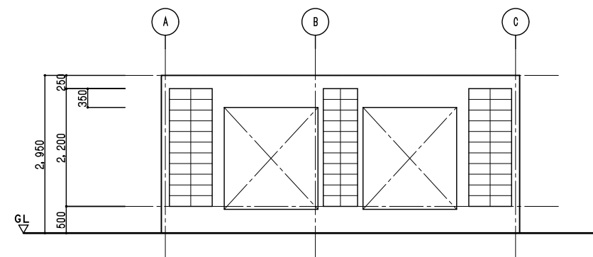
2通ブロック割図 S=1/50
