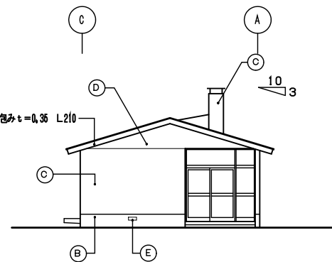
東立面図 S=1/100
