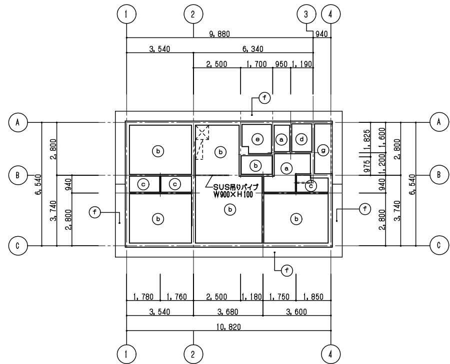
天井伏図 S=1/100
