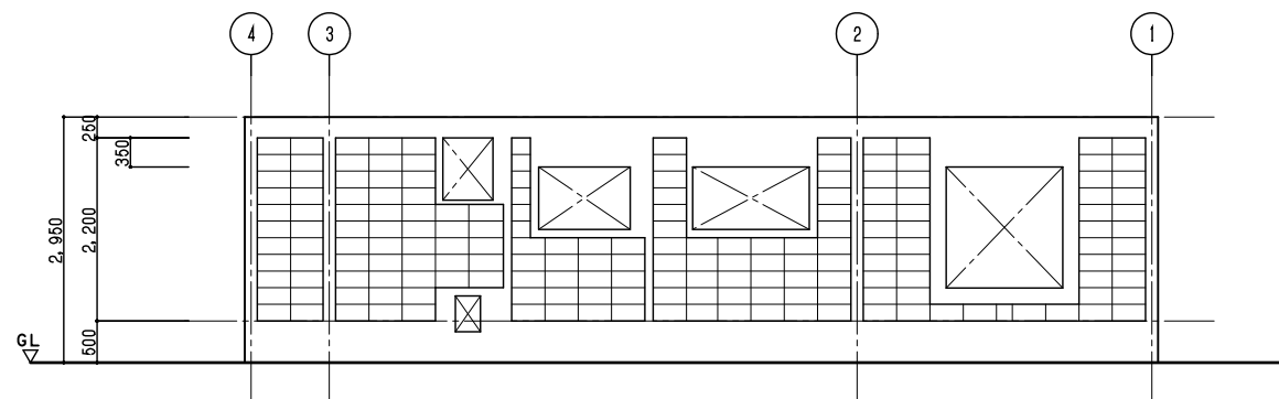
A通ブロック割図 S=1/50
