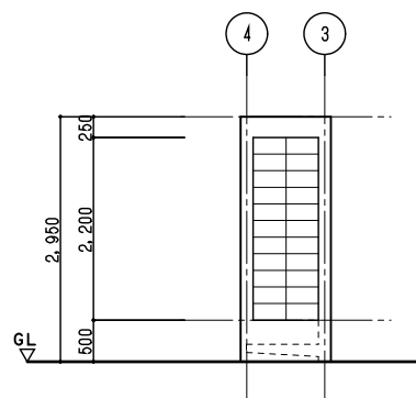
B通ブロック割図 S=1/50
