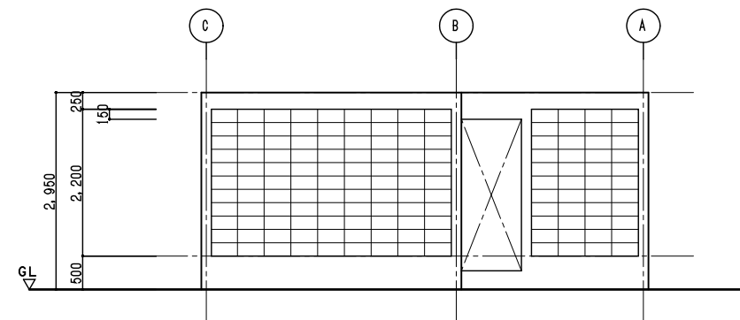
3通・4通ブロック割図 S=1/50
