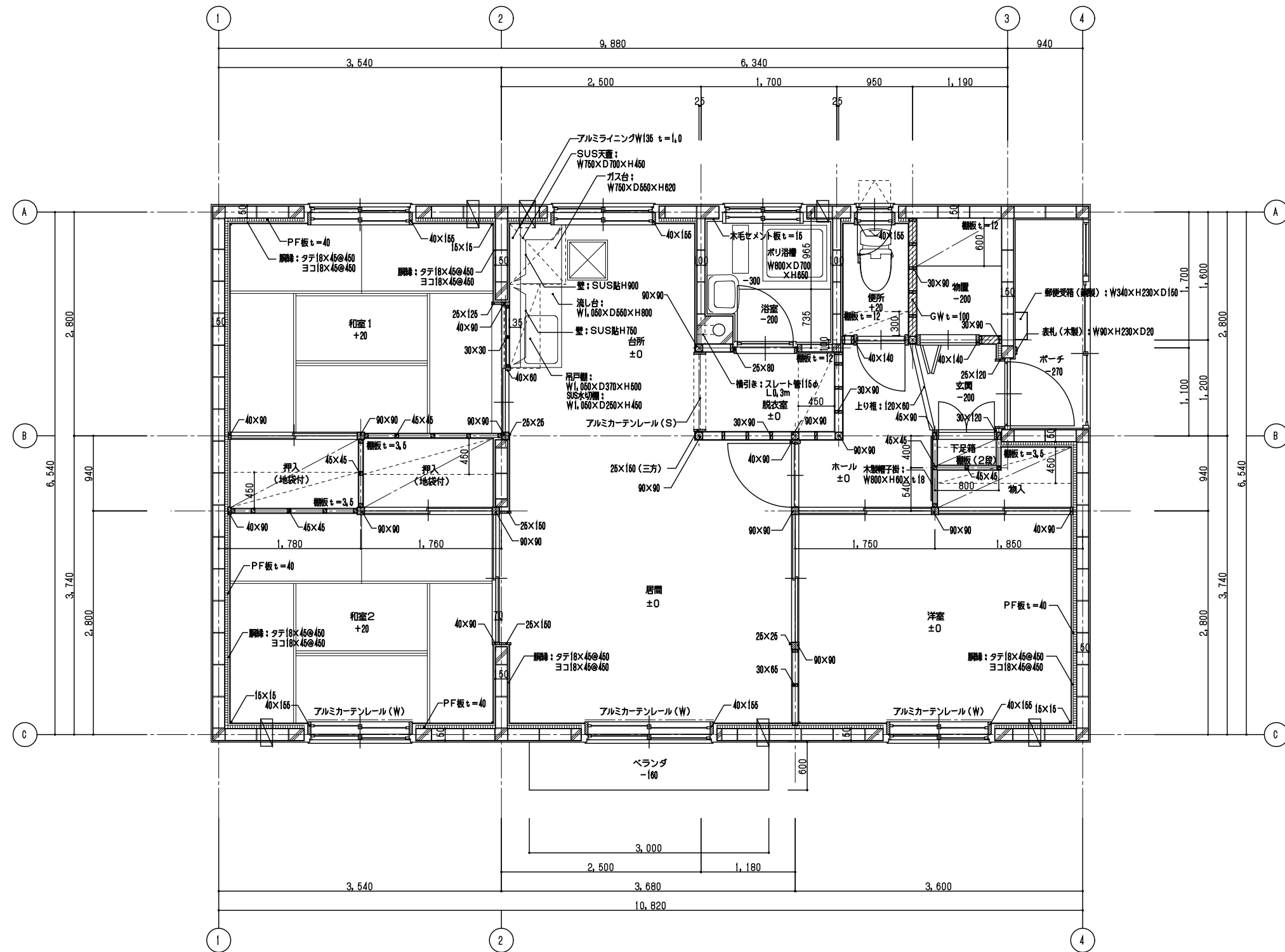
平面詳細図 S=1/30
