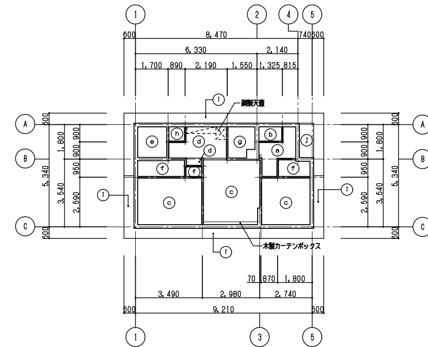
天井伏図 S=1/100
