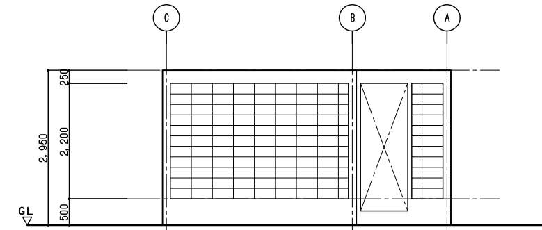
4通・5通ブロック割図 S=1/50
