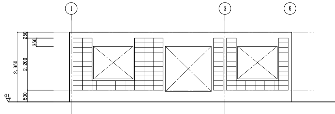
C通ブロック割図 S=1/50
