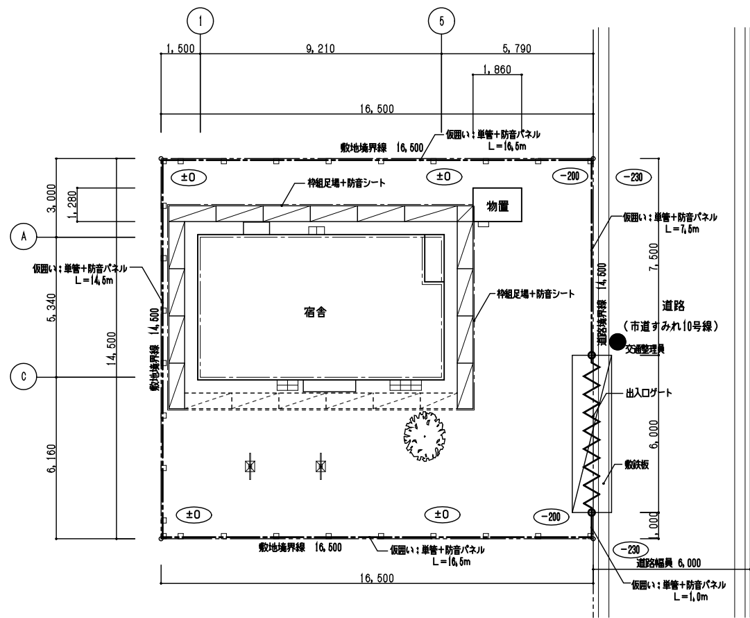
仮設計画図 S=1/100
