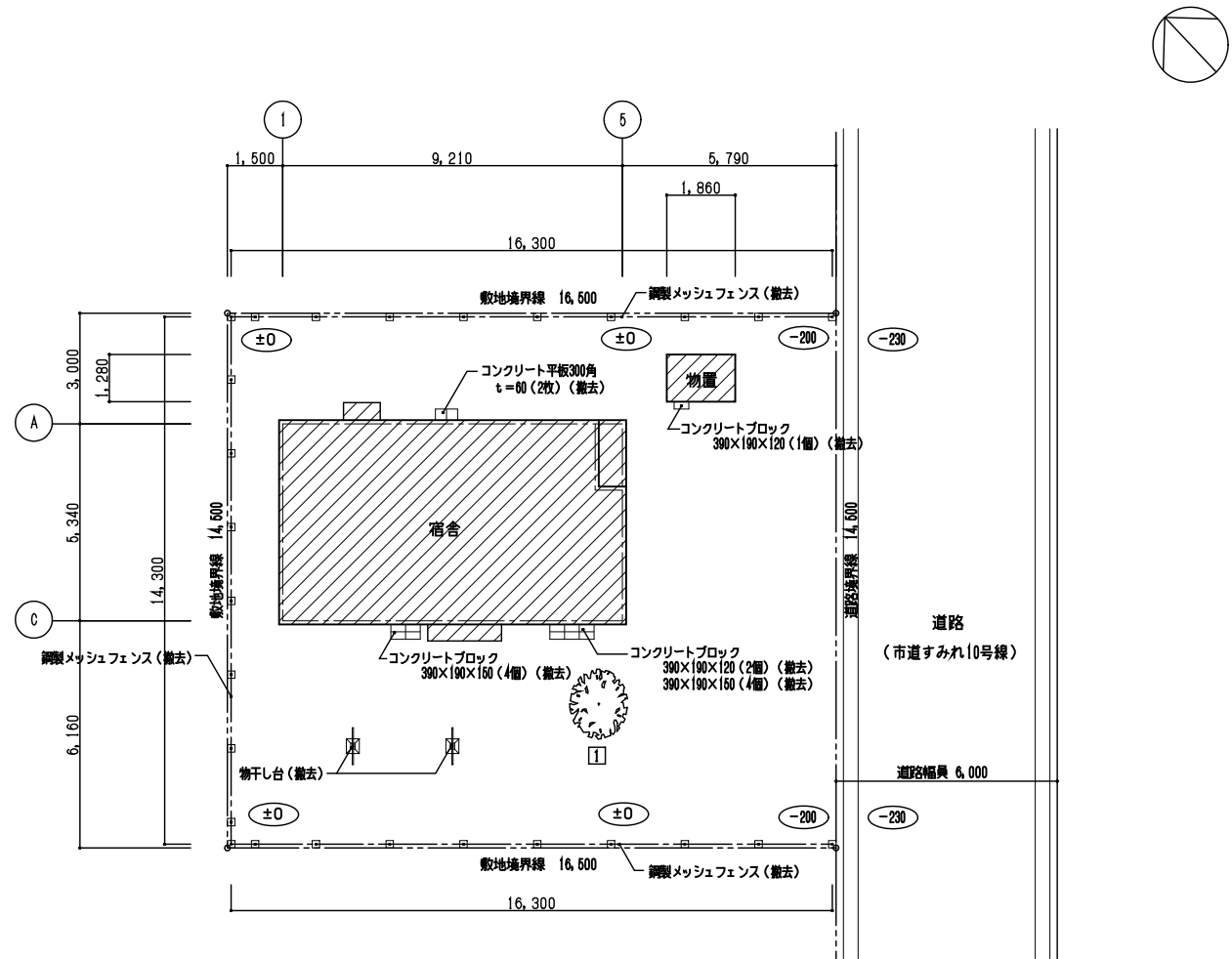
外構図 S=1/100
