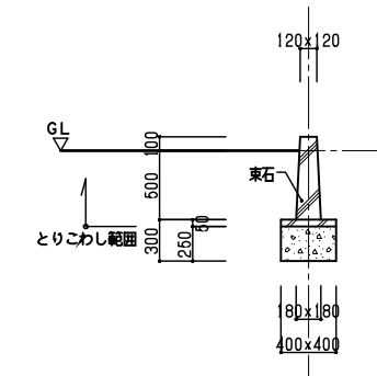
束石 S=1/30
