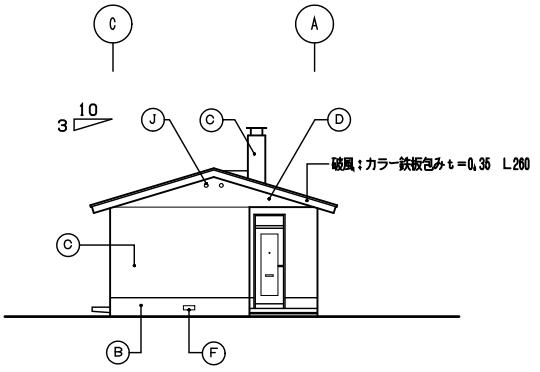
西立面図 S=1/100
