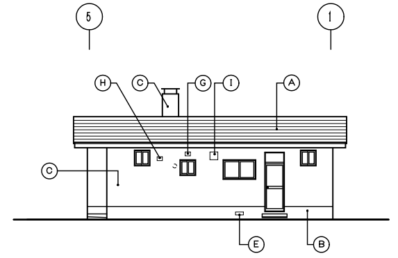
北立面図 S=1/100
