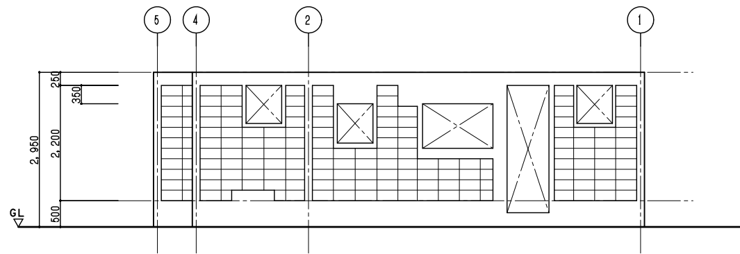
A通・B通ブロック割図 S=1/50
