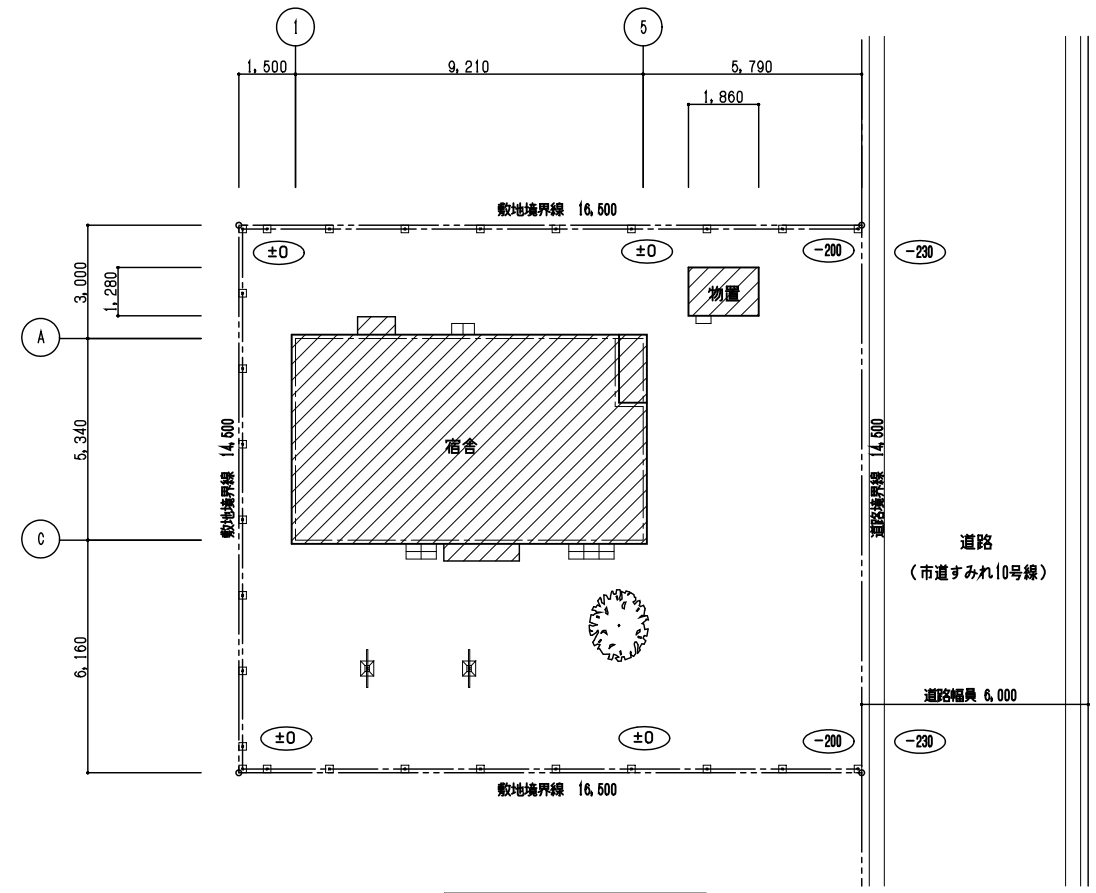
配置図 S=1/100
