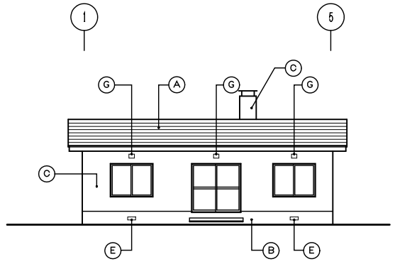
南立面図 S=1/100
