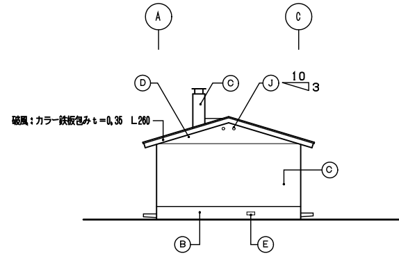
東立面図 S=1/100
