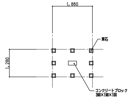
基礎伏図 S=1/50
