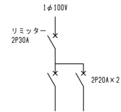
分電盤結線図
