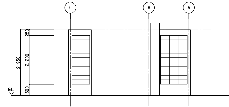
2通・3通ブロック割図 S=1/50
