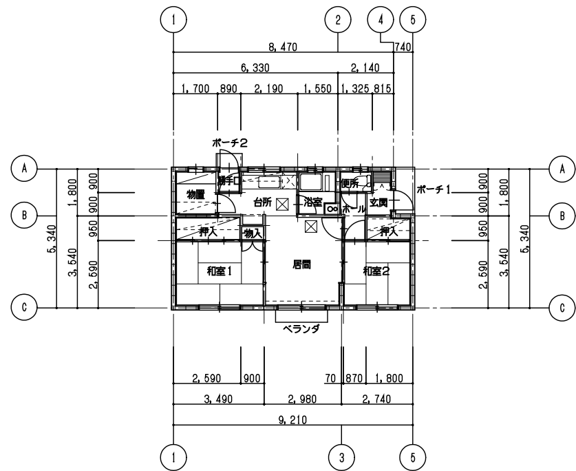
平面図 S=1/100
