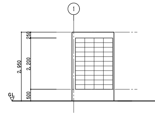
B通帳壁ブロック割図 S=1/50
