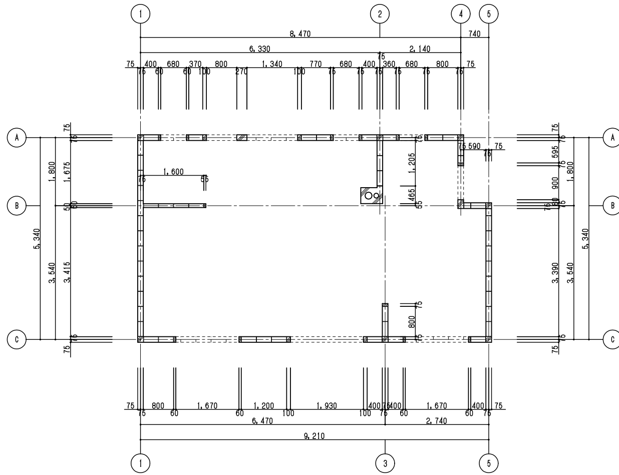
ブロック割平面図 S=1/50
