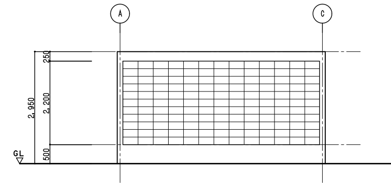
1通ブロック割図 S=1/50
