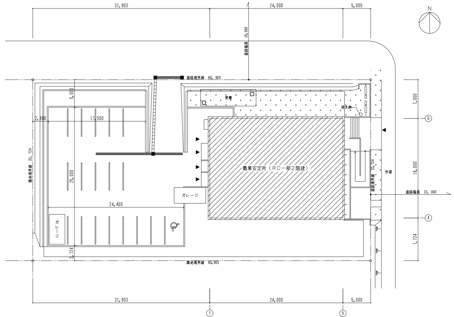
配置図 S=1/200
