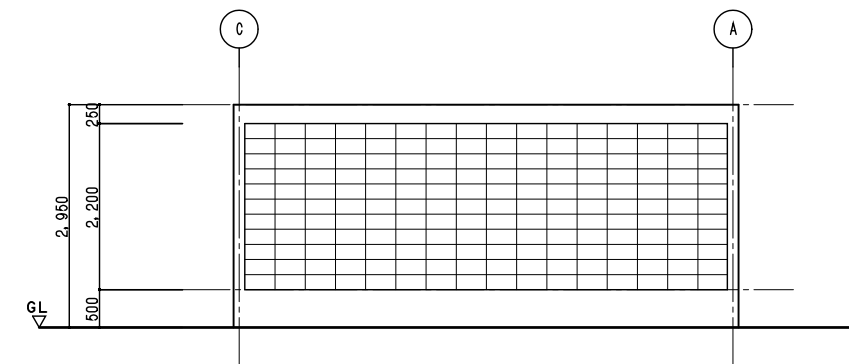
4通ブロック割図 S=1/50
