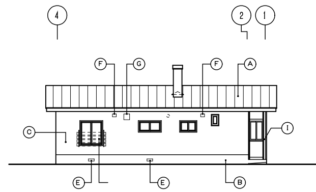
北立面図 S=1/100
