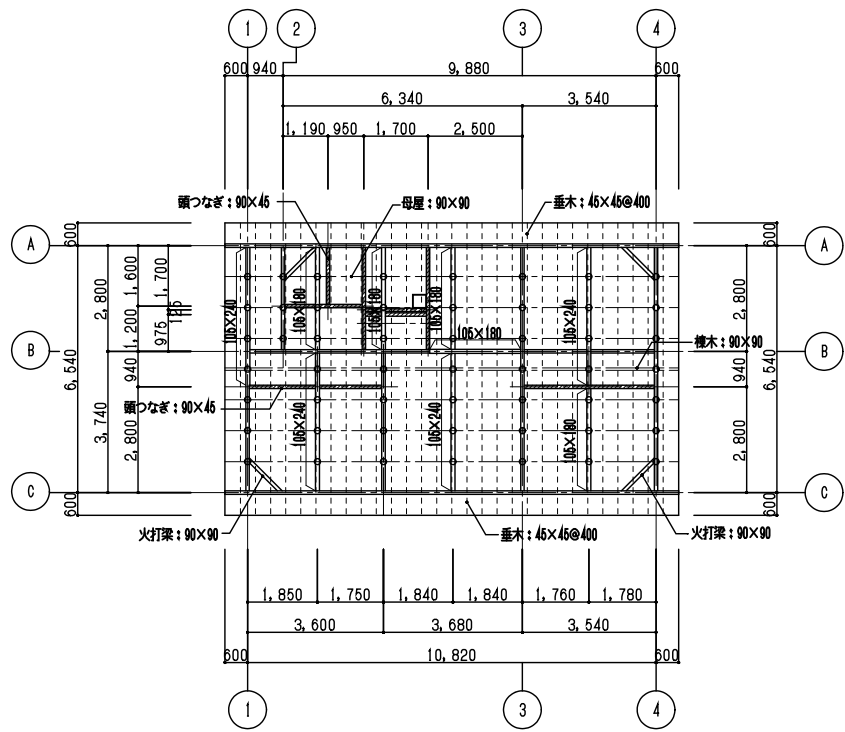
小屋伏図 S=1/100
