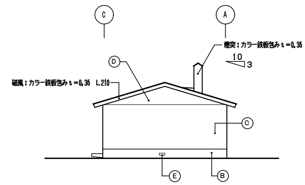
東立面図 S=1/100
