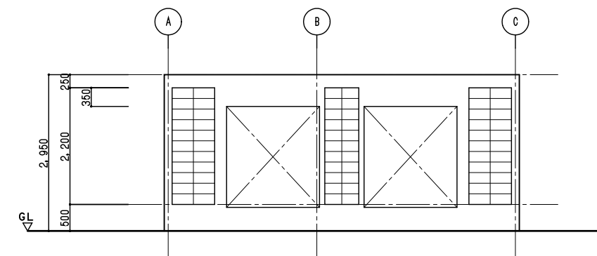
3通ブロック割図 S=1/50
