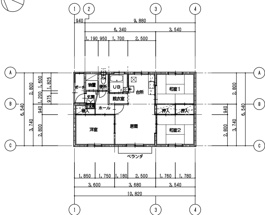
平面図 S=1/100
