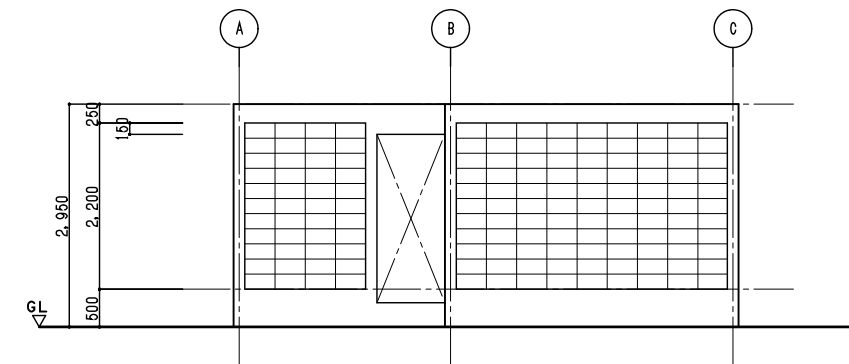
1通・2通ブロック割図 S=1/50
