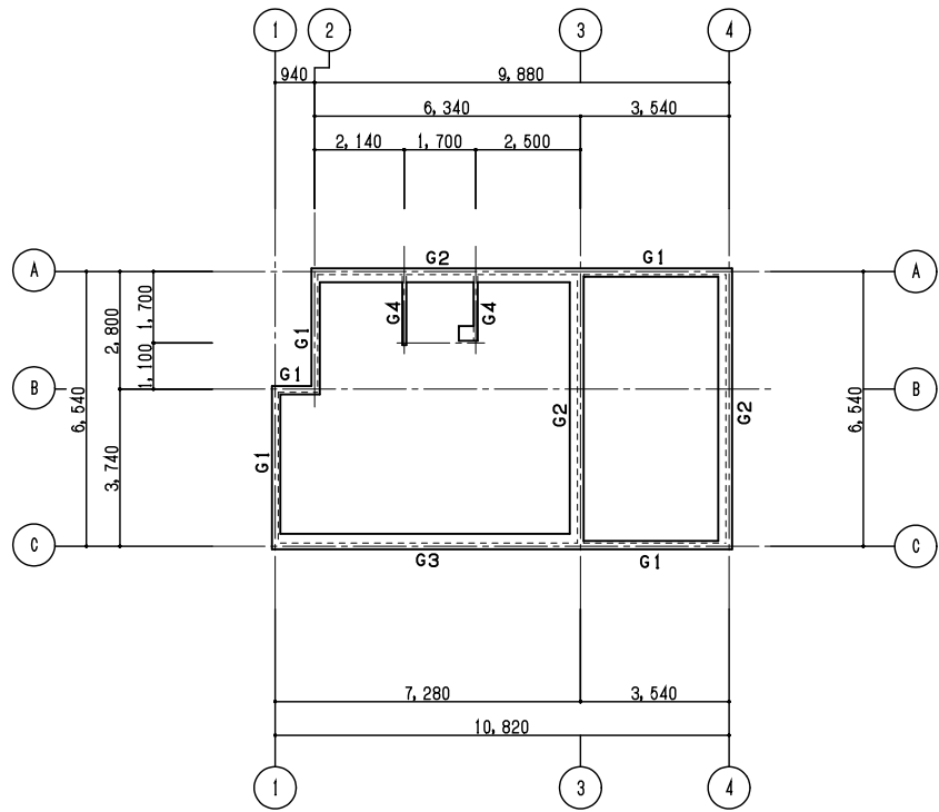
臥梁伏図 S=1/100
