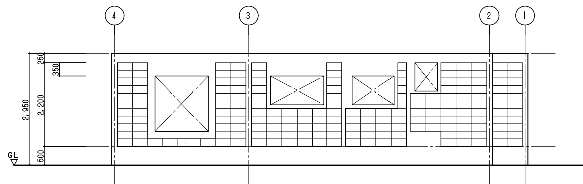
A通・B通ブロック割図 S=1/50
