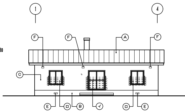
南立面図 S=1/100
