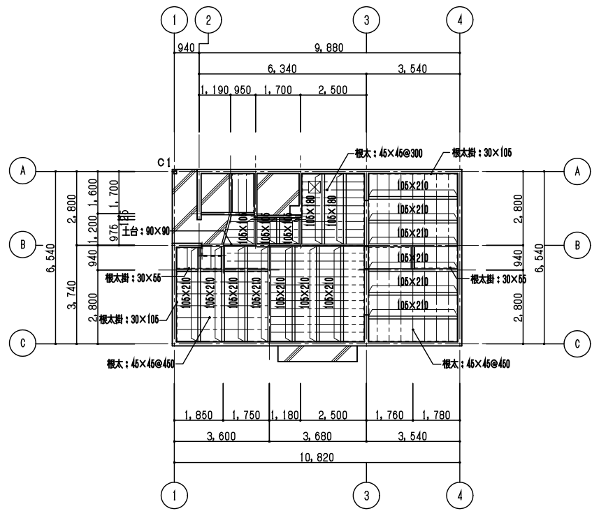
床伏図 S=1/100
