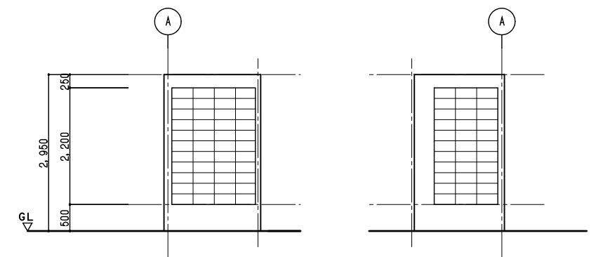
浴室廻りブロック割図 S=1/50
