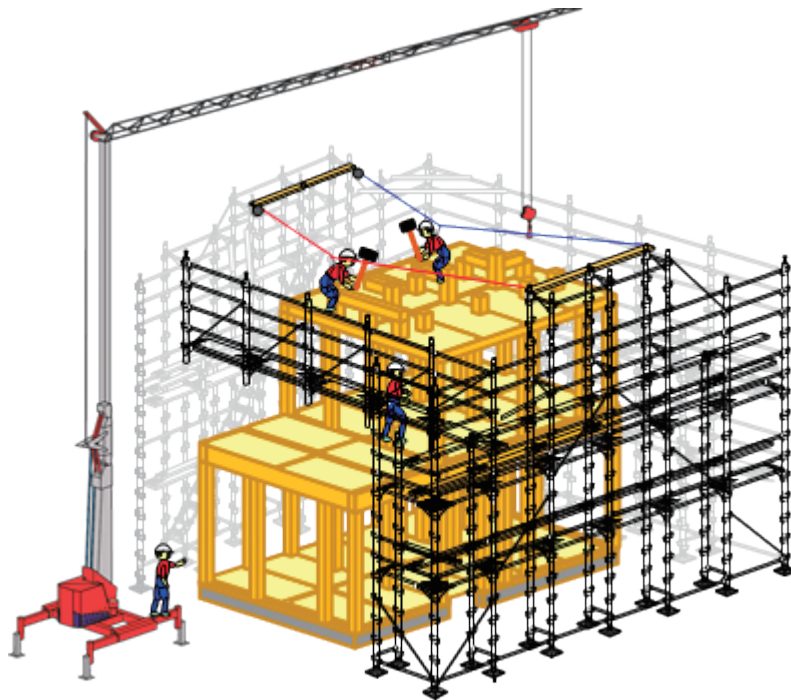
図2-27 本足場（二側足場）
