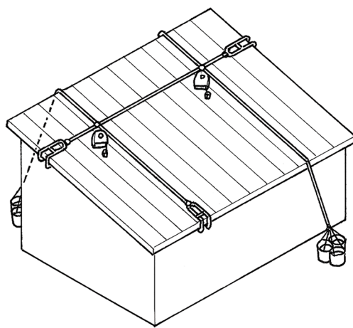
図2-35 片流れ屋根の親綱等設置の例
