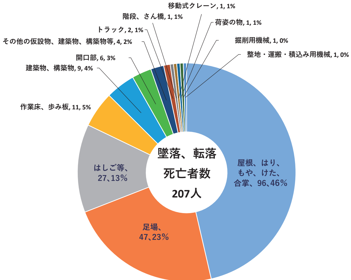
図1-3 木建工事における墜落・転落災害（死亡）の起因物（小分類）発生状況 (平成25年～令和4年累計)
