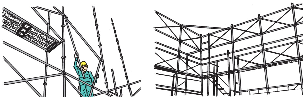
図2-13 手すり先行部材例
