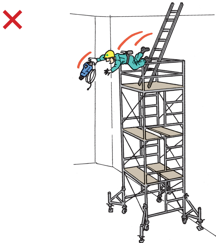
図3-10 移動式足場上ではしごを使用しない
