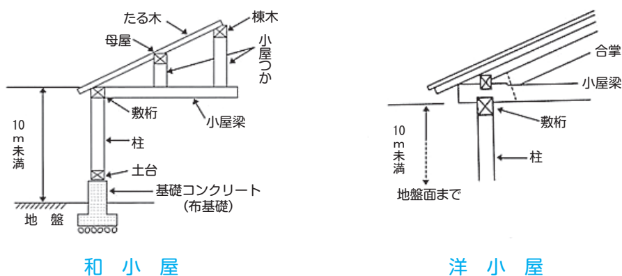
図2-10 ガイドラインが適用される工事例
