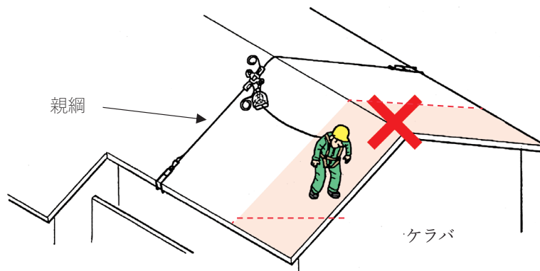
図2-42 作業範囲
