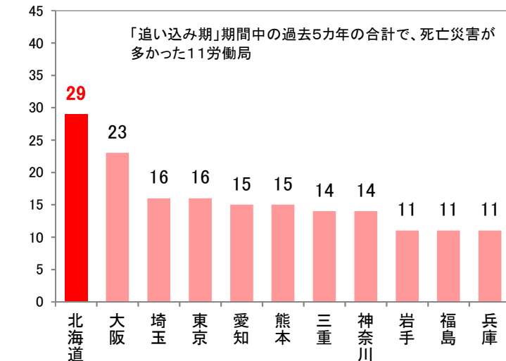
建設業における都道府県労働局別死亡災害発生状況 平成29年～令和3年（各年10月～12月）
