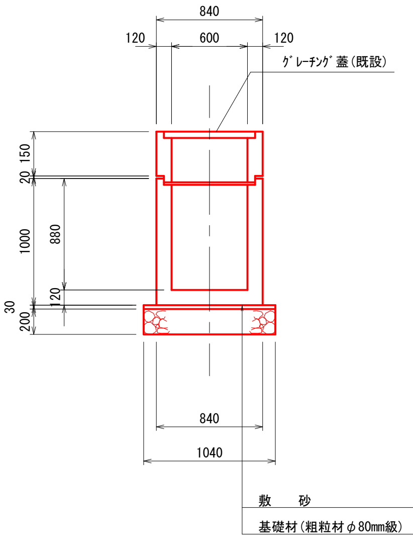
標準図 S=1:30 集水桝 I 型A 撤去・再設置
