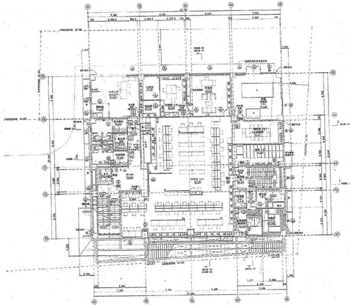
2階平面図 1/100
