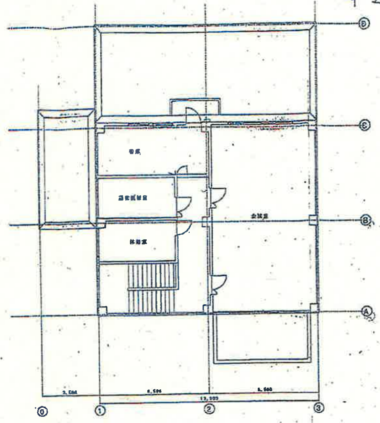
2階平面図 1/100
