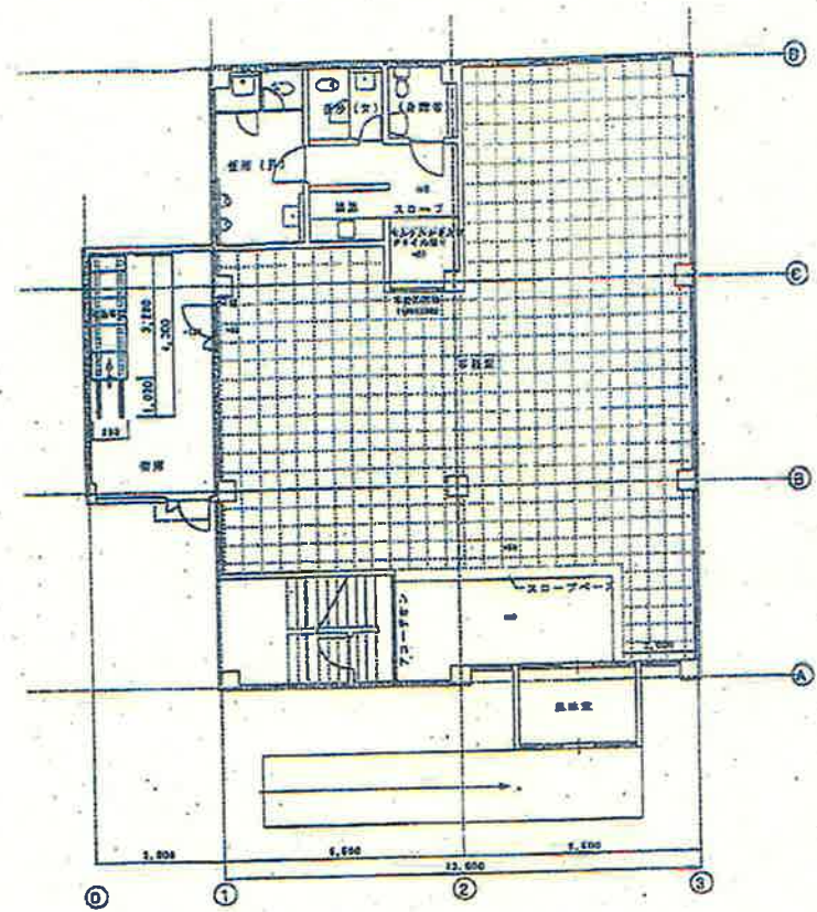
1階平面図 1/100
