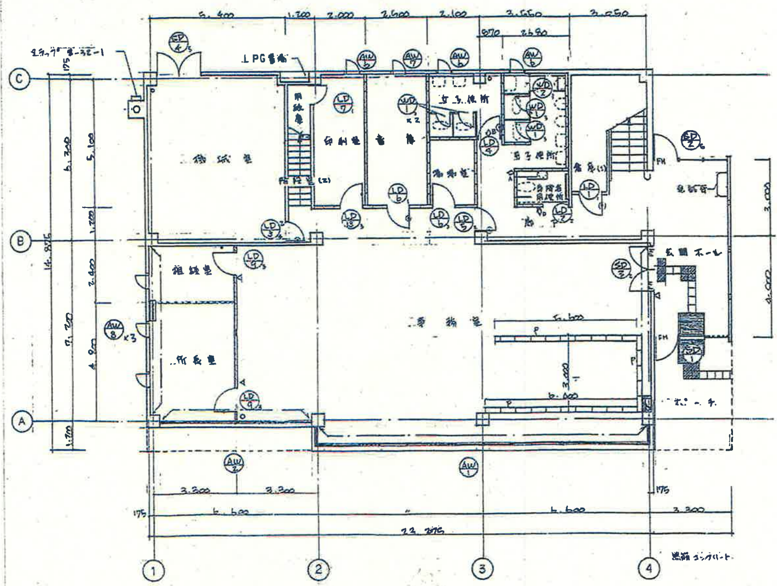
1階平面図
