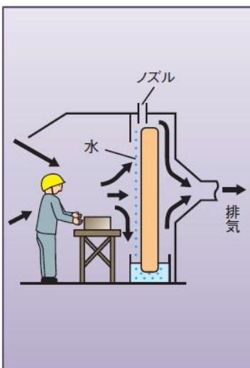
局所排気装置(囲い式)の例
