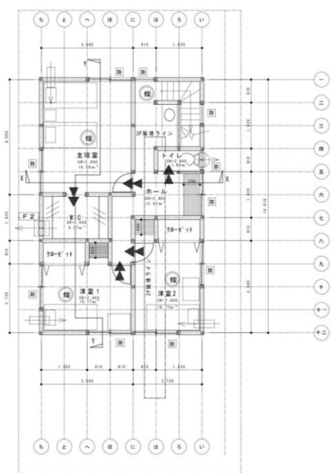
2階平面詳細図 S=1/100
