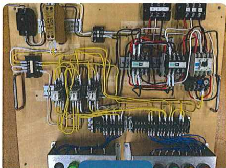
制御回路
