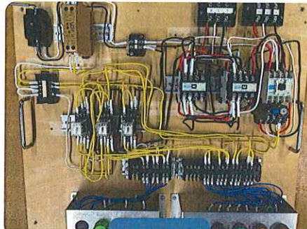
制御回路
