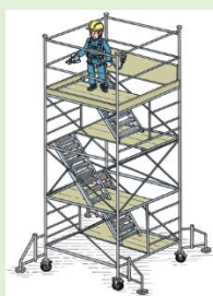
ローリングタワー (移動式足場)
