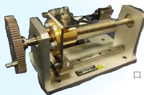
ダブルピンゼネバ
