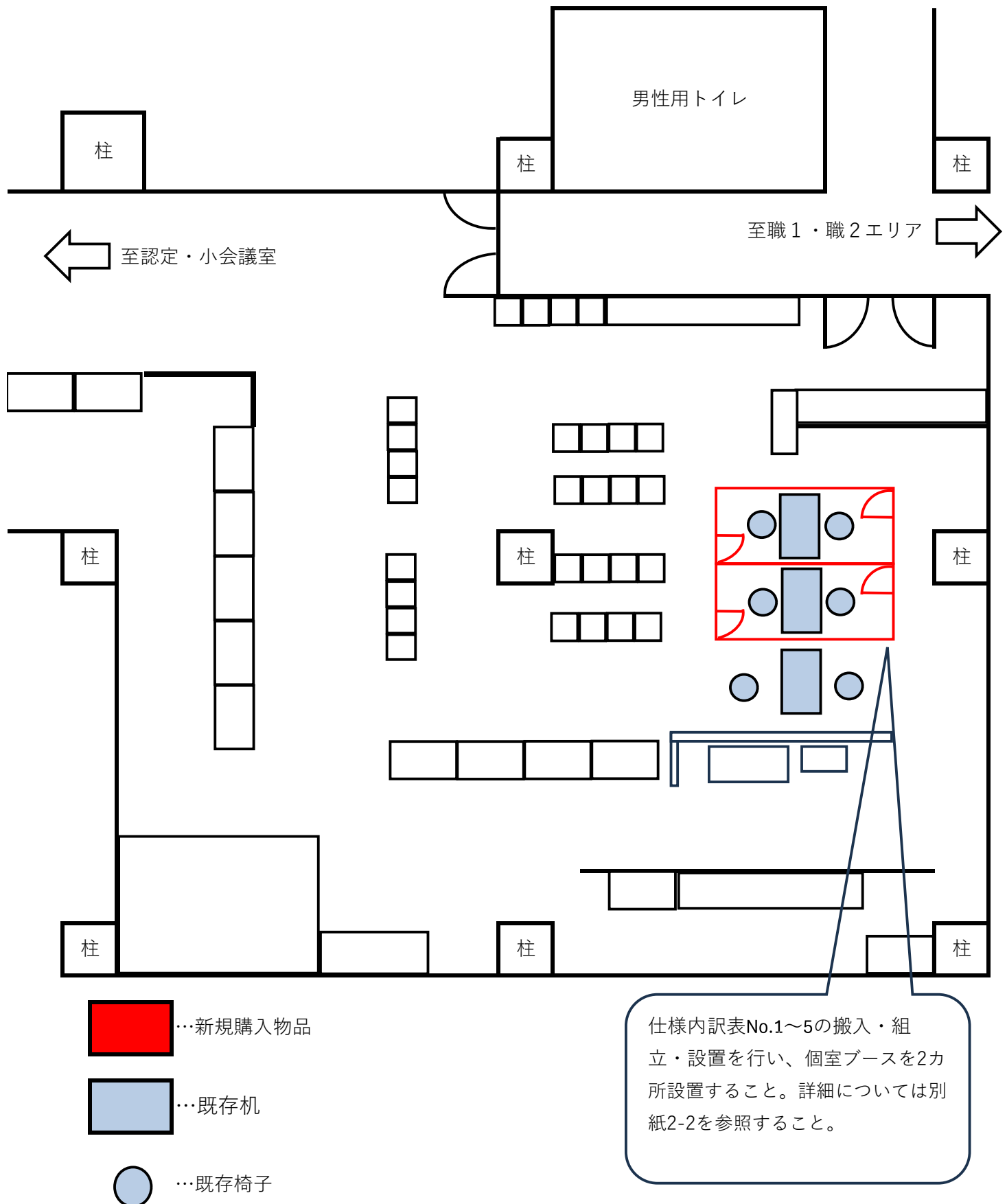
松戸所3階（給付課資格決定エリア） 変更後レイアウト図
