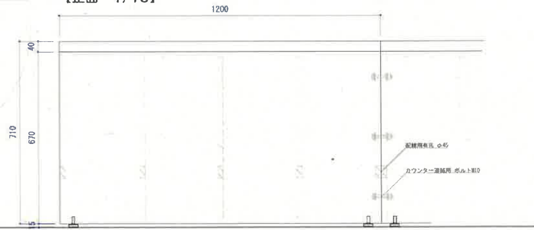
【正面 1/10】
