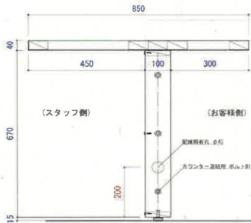
【側断面 1/10】
