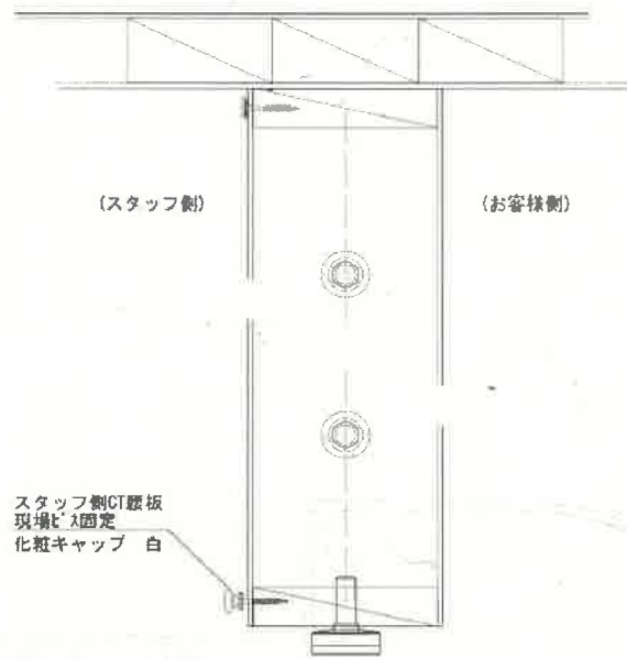
【側断面 1/10】
