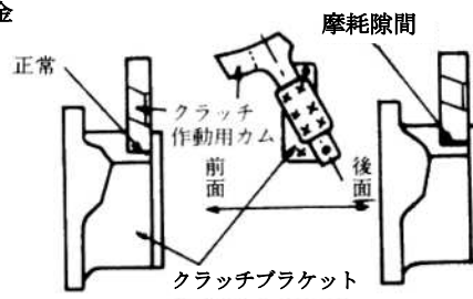
摩耗隙間とは、クラッチブラケットとクラッチ作用カムのスライド部との隙間をいう。
